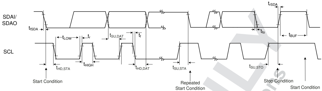
图 8-1. I²C Timings
