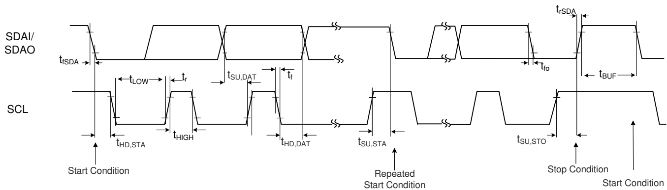
图 31. I²C Timings
