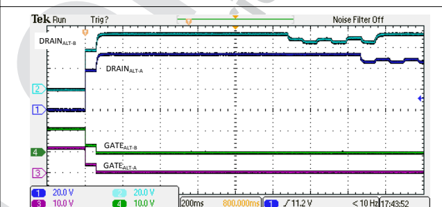
10-7. 4-Pair Backoff Due to I_{LIM} Fault
