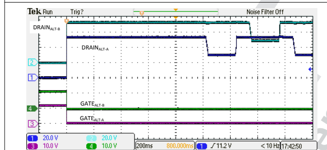
FIG 10-8. 4-Pair Backoff Due to 4PPCut Fault
