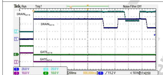
10-8. 4-Pair Backoff Due to 4PPCut Fault
