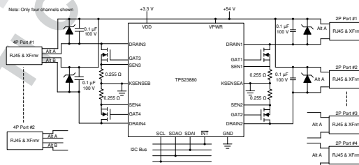
概略回路図
