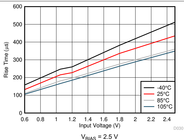
図 6-43. Rise Time vs Input Voltage
