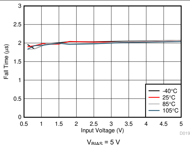
図 6-22. Fall Time vs Input Voltage
