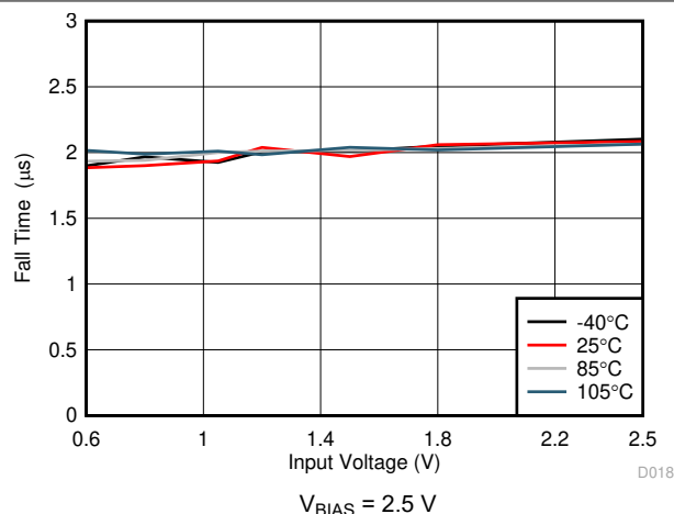
図 6-21. Fall Time vs Input Voltage
