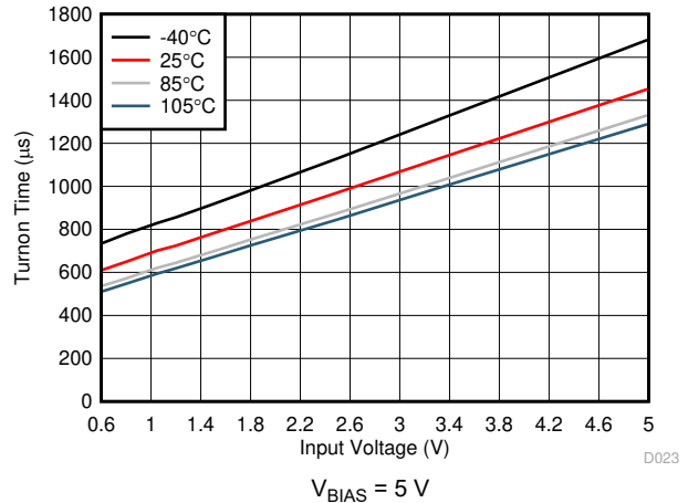
6-28. Turnon Time vs Input Voltage
