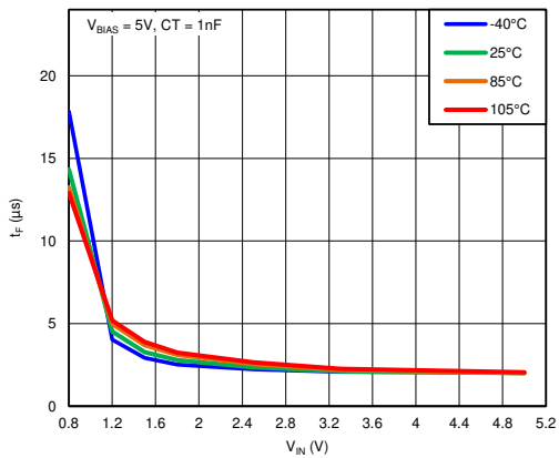
FIG 15. t_F vs. V_{IN} ( V_{BIAS} = 5\text{ V} , C_T = 1\text{ nF} )
