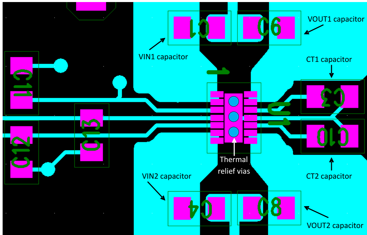
图 37. Layout Example
