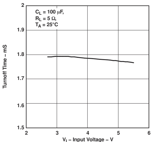
図 6-20. TURNOFF TIME vs INPUT VOLTAGE
