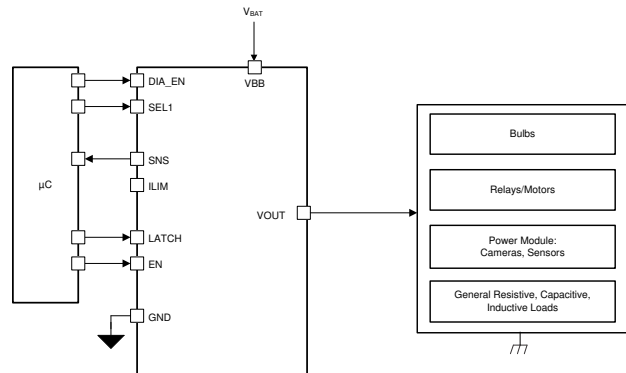
概略回路図
