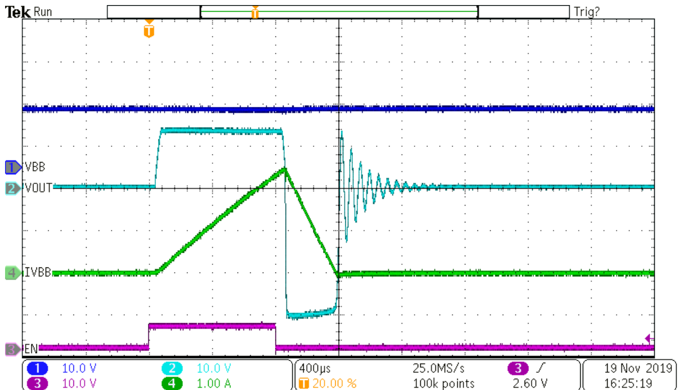
✎ 9-3. TPS1HB50-Q1 Inductive Discharge (5 mH)
