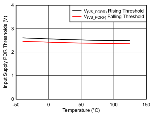
5-9. Input Supply POR Thresholds vs Temperature
