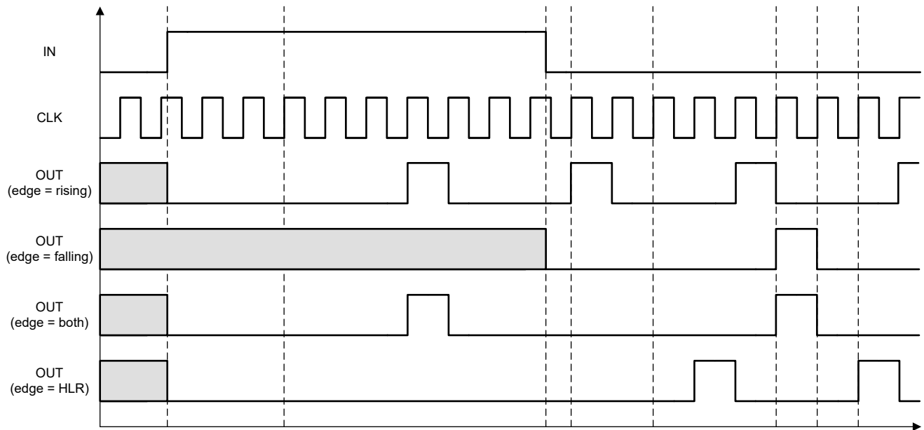
図 7-15. カウンタ出力タイミングの例 (DATA = 3)
