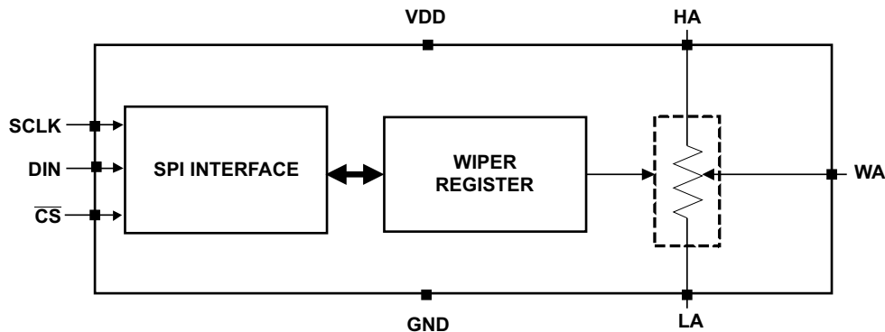
概略回路図
