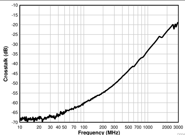
图 7-2. SBU Crosstalk
