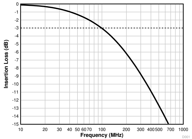
图 7-16. CC Bandwidth
