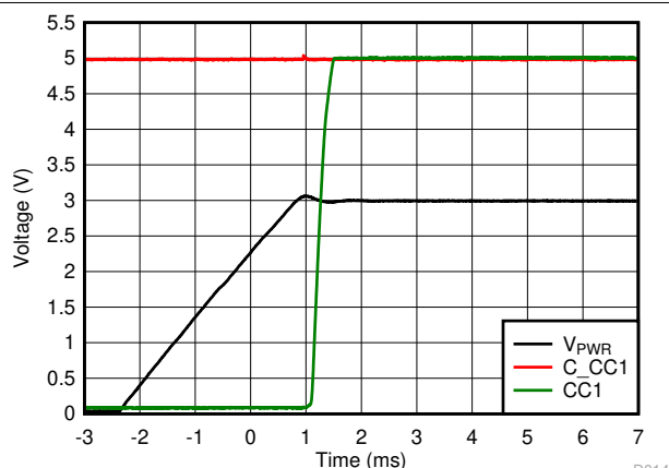
FIG 7-27. CC FET Turnon Timing
