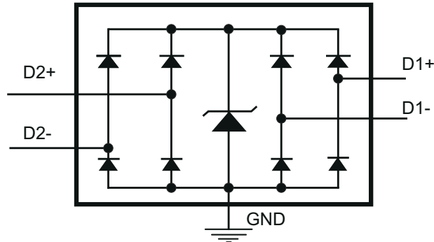
7-1. TPD4EUSB30 Circuit
