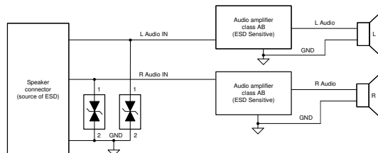
代表的なアプリケーション回路図
