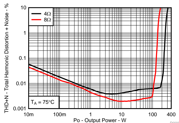
全高調波歪み
