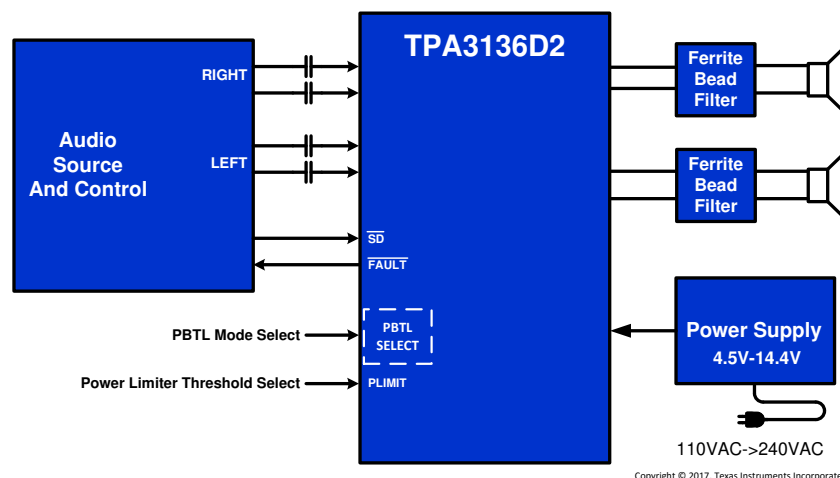
概略回路図
