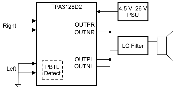
図 34. PBTL Mode
