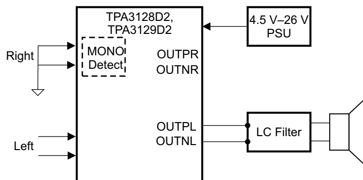
図 35. MONO Mode
