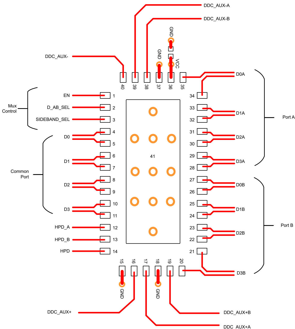
図 8-6. Layout Example
