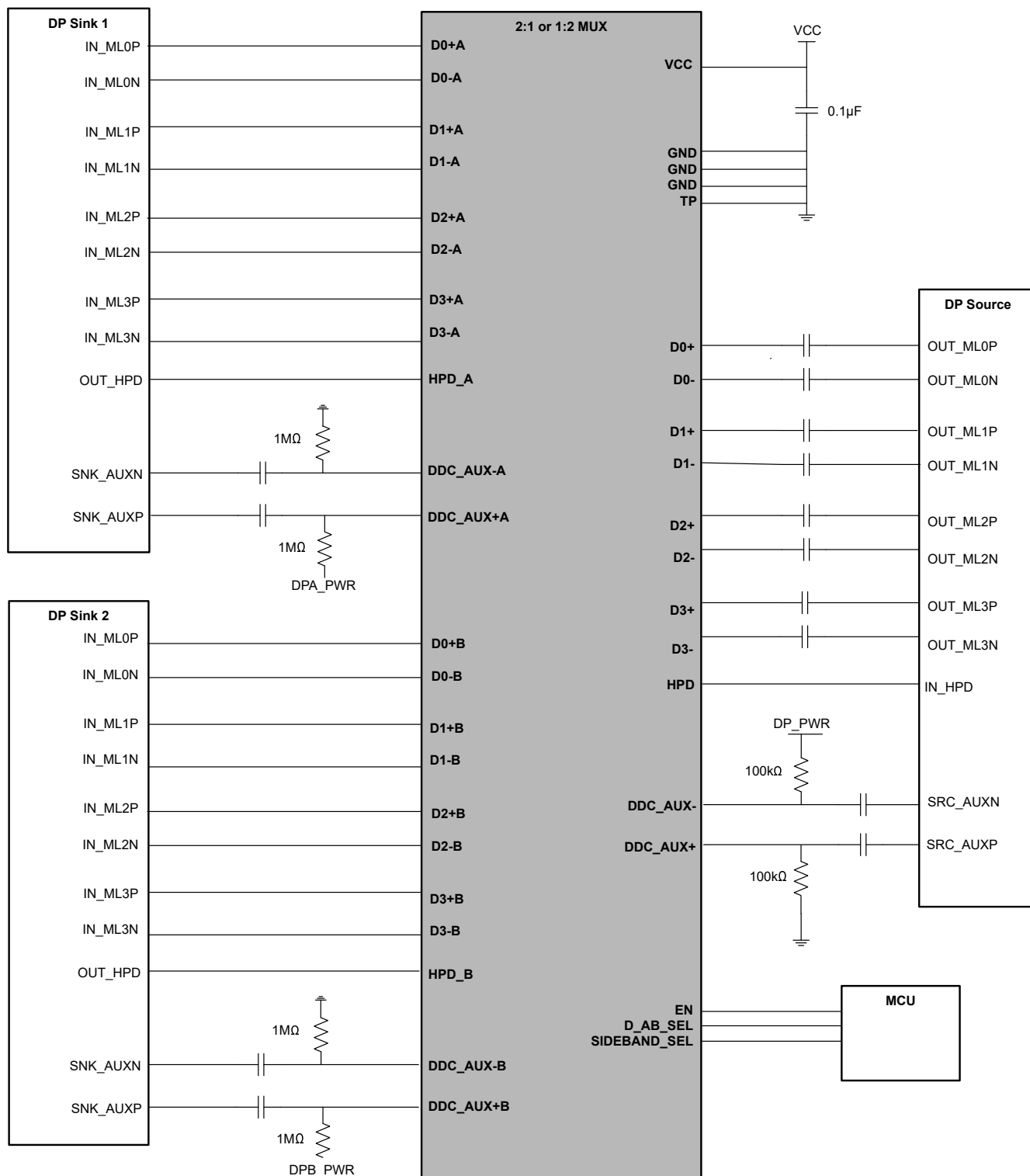
8-8. DisplayPort 1:2 Switching
