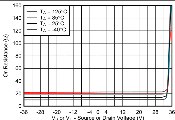
図 6-1. オン抵抗とソースまたはドレイン電圧との関係
