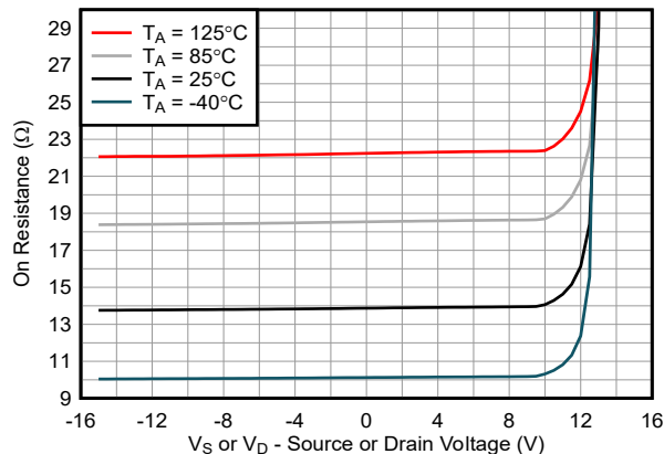
図 6-3. オン抵抗とソースまたはドレイン電圧との関係
