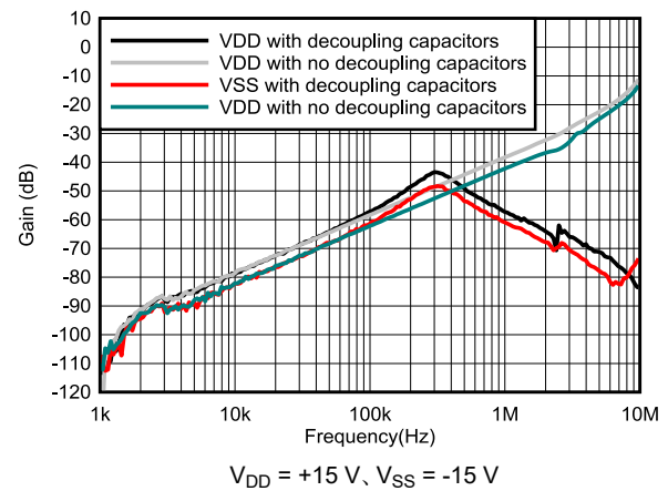
図 5-24. ACPSRR と周波数との関係
