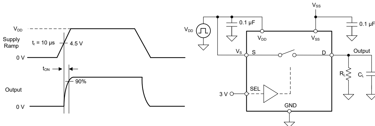
図 6-5. t_{ON}(V_{DD}) 時間の測定に使用する構成
