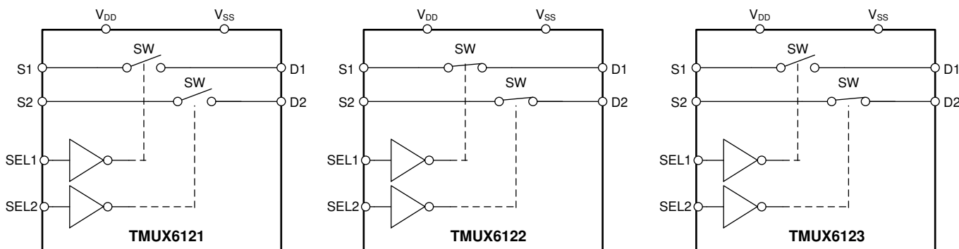
概略回路図
