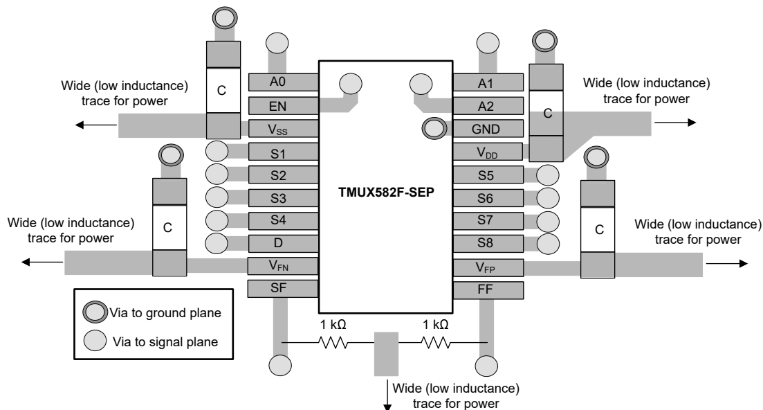
図 9-3. TMUX582F-SEP PW Layout Example
