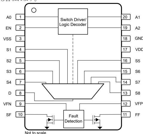
概略回路図
