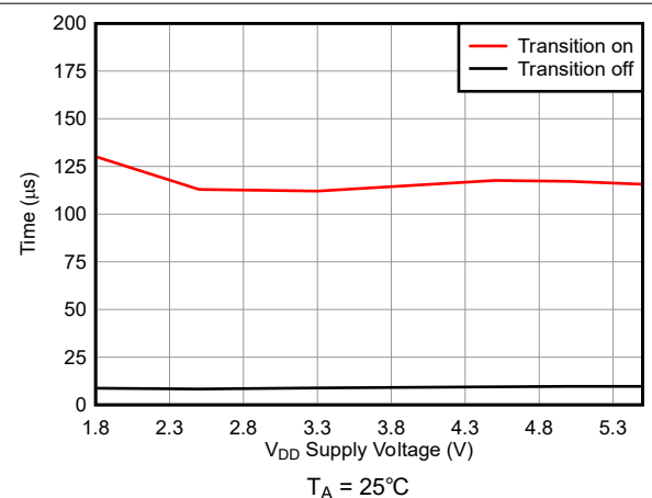
図 5-11. 遷移時間と電源電圧との関係
