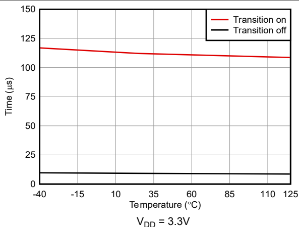
図 5-10. サンプリング時間と温度との関係
