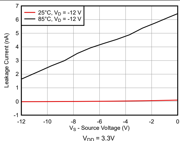
図 5-4. ISOFF リークとソース電圧との関係
