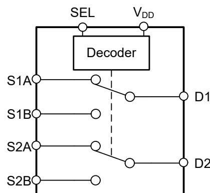
TMUX4827 ブロック図
