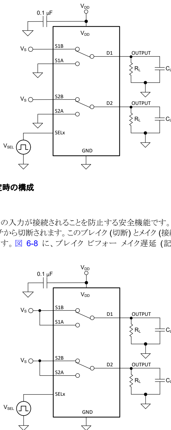
図 6-8. ブレイク ビフォー メイク遅延測定時の構成
