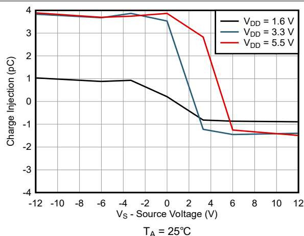
図 5-13. 電荷注入とソース電圧との関係
