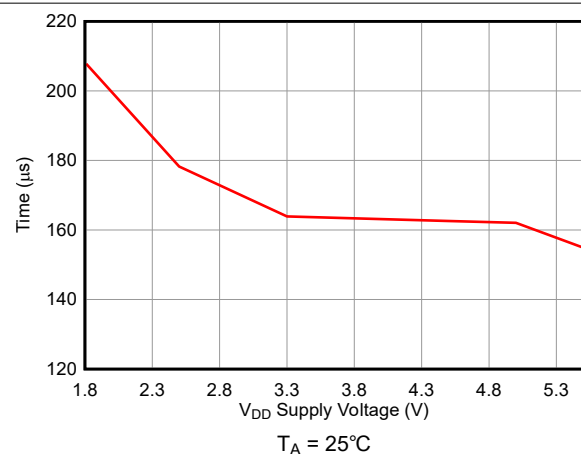
図 5-12. tBBM と電源電圧との関係
