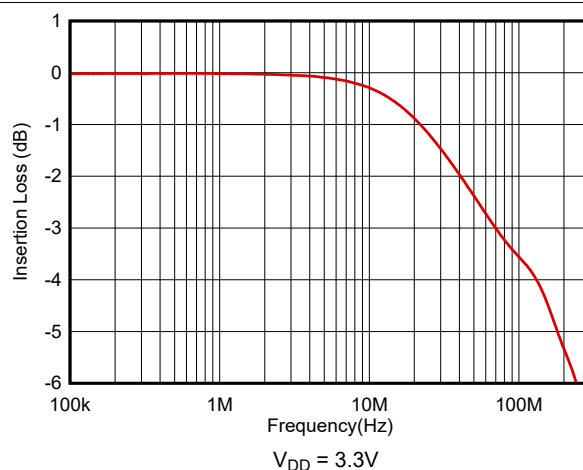
図 5-18. 挿入損失と周波数との関係
