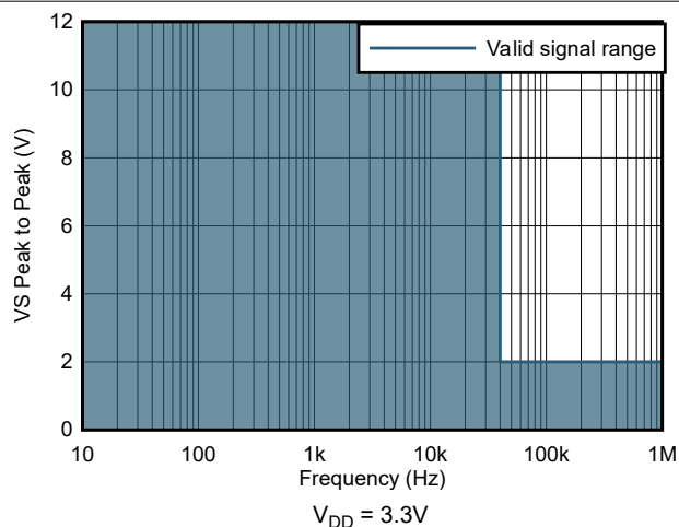
図 5-22. 最大信号スイング
