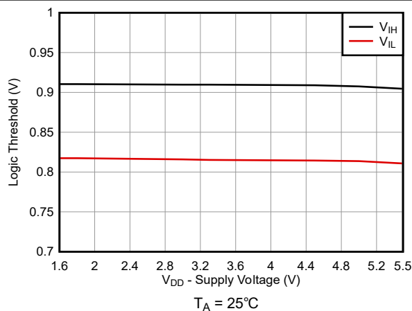
図 5-9. ロジック スレッシュホルドと電源電圧との関係
