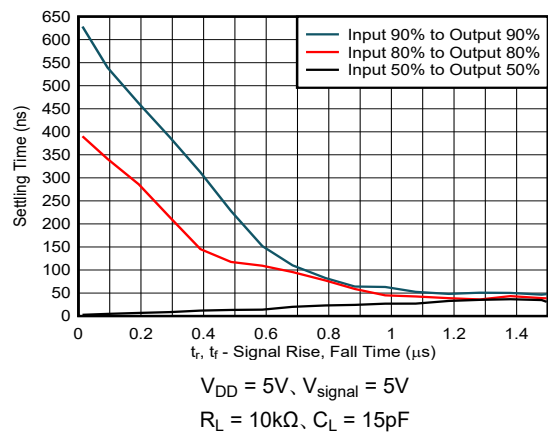
図 6-6. システムのセtring タイム
