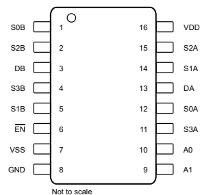
図 5-5. TMUX4052 (DYY パッケージ)、16 ピン SOT-23-THIN (上面図)
