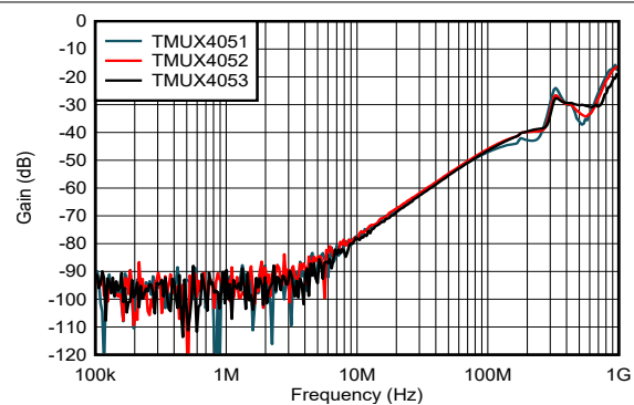
図 6-8. オフ絶縁と周波数との関係
