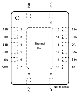
図 5-6. TMUX4052 (BQB パッケージ)、16 ピン WQFN (上面図)
