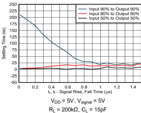
図 6-5. システムのセtring タイム
