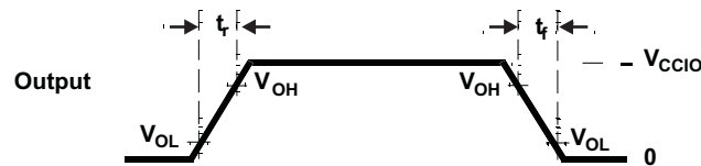
图 6-2. CMOS-Level Outputs
