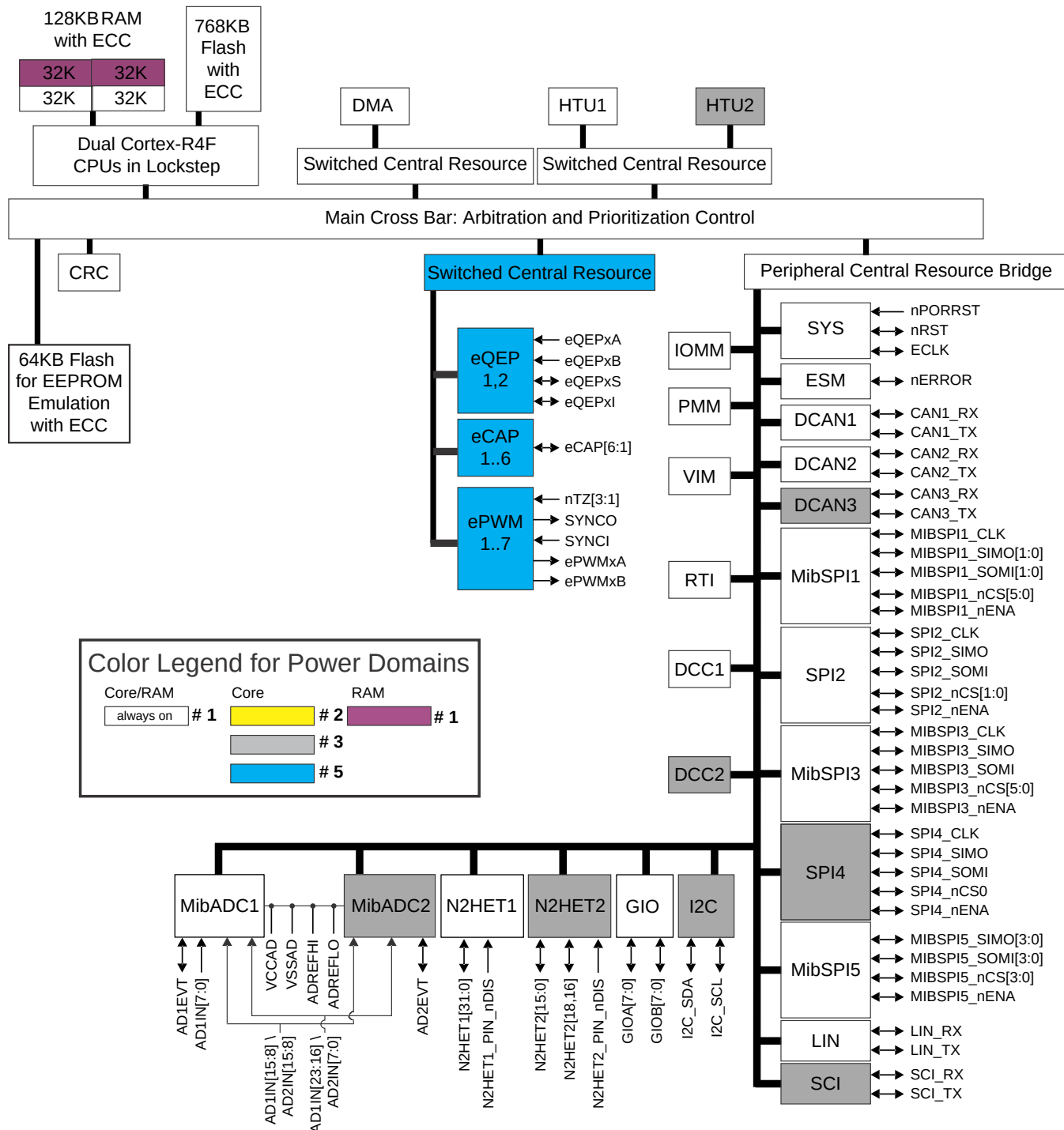
図 1-1. 機能ブロック図
