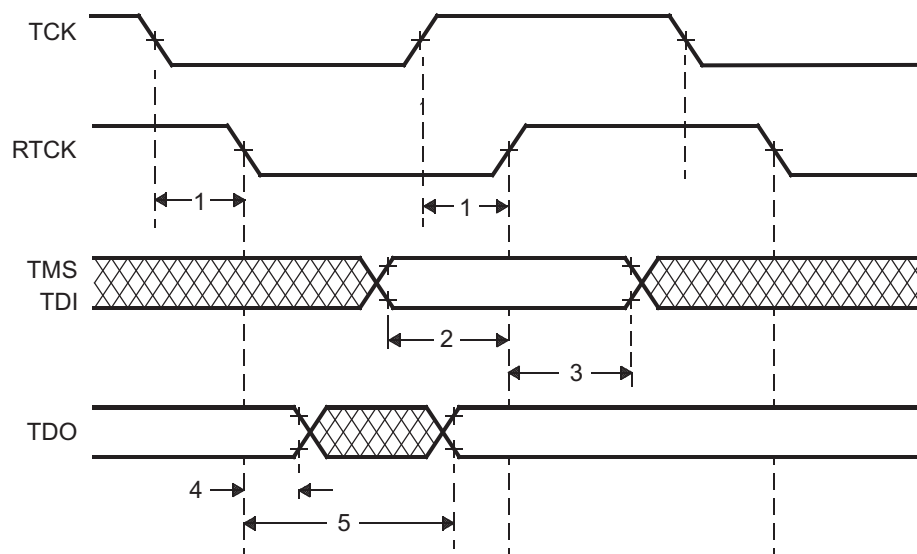
図 5-15. JTAG Timing
