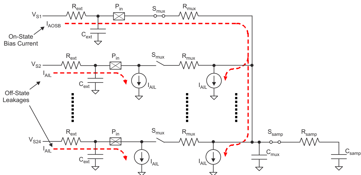
図 8-11. MibADC Input Equivalent Circuit
