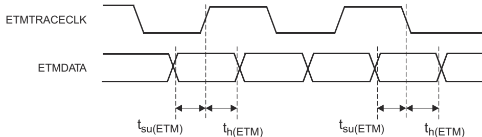
図 7-31. ETMDATA Timing
