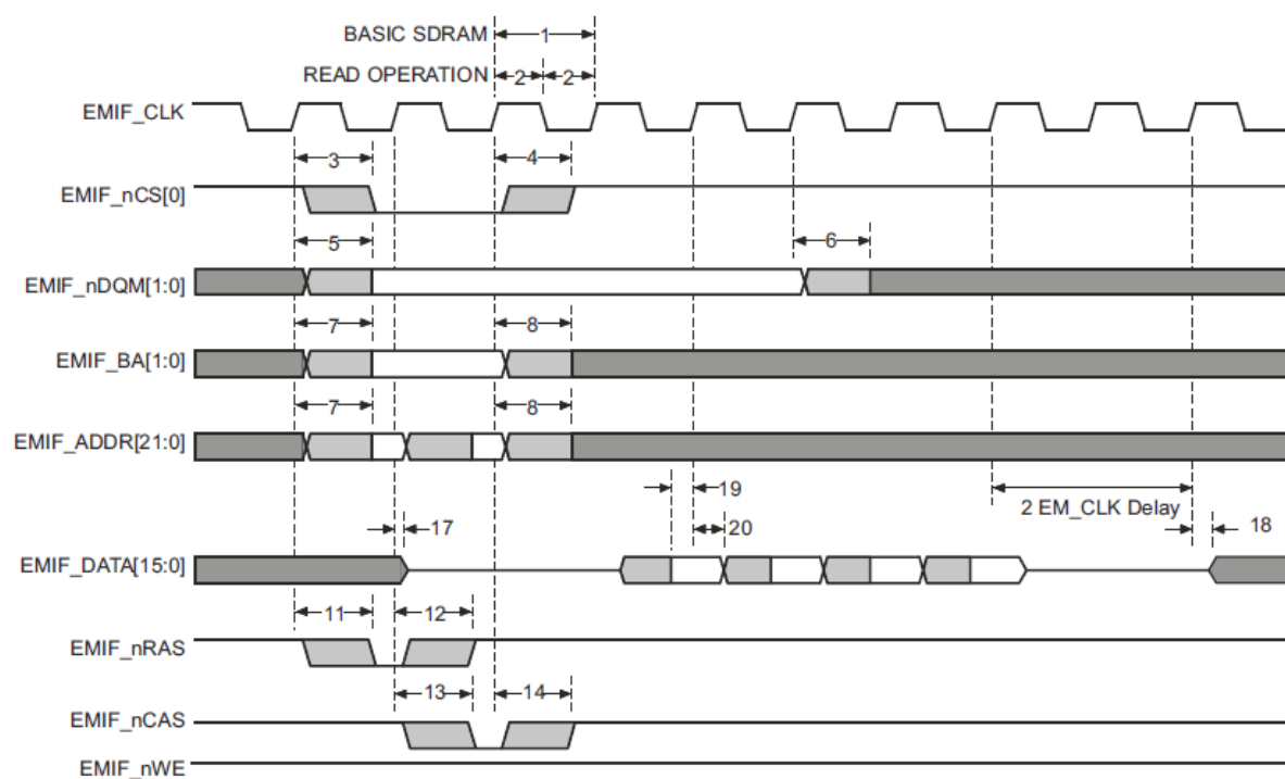
図 4-15 基本 SDRAM リード動作
