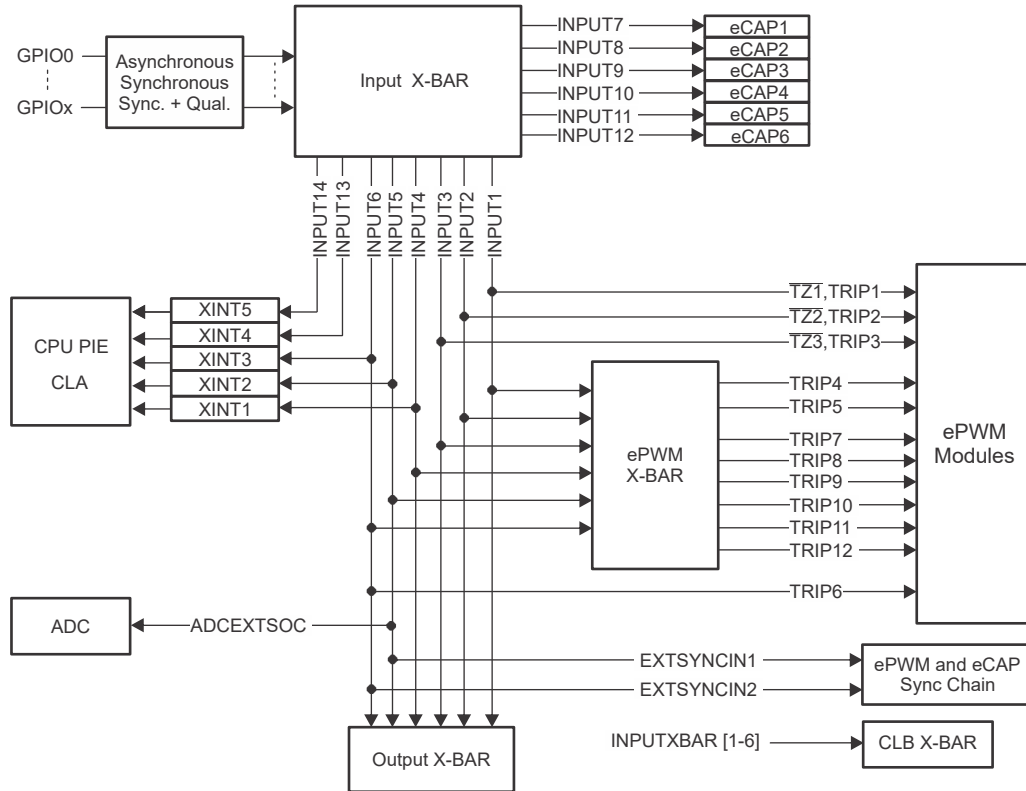
図 5-7. 入力クロスバー
