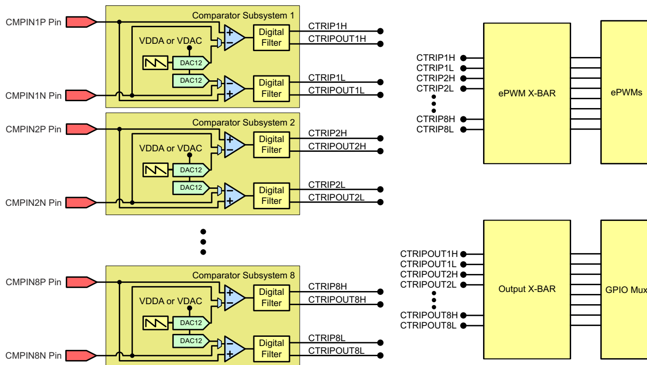
図 6-41. CMPSS 接続 (337 ボール ZWT および 176 ピン PTP)
