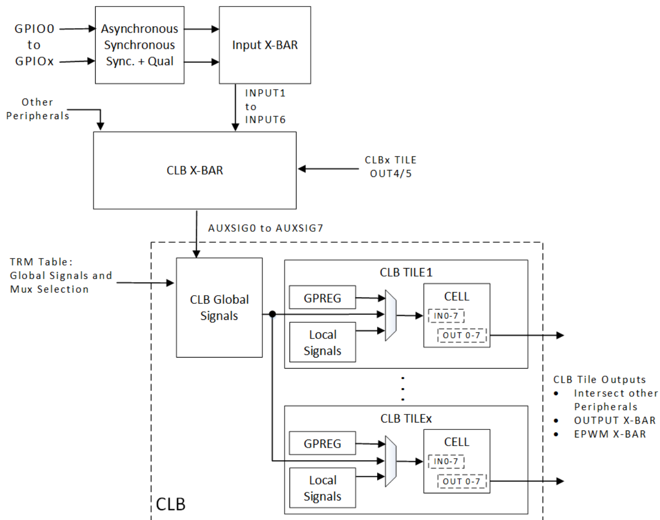
図 7-5. CLB の概要
