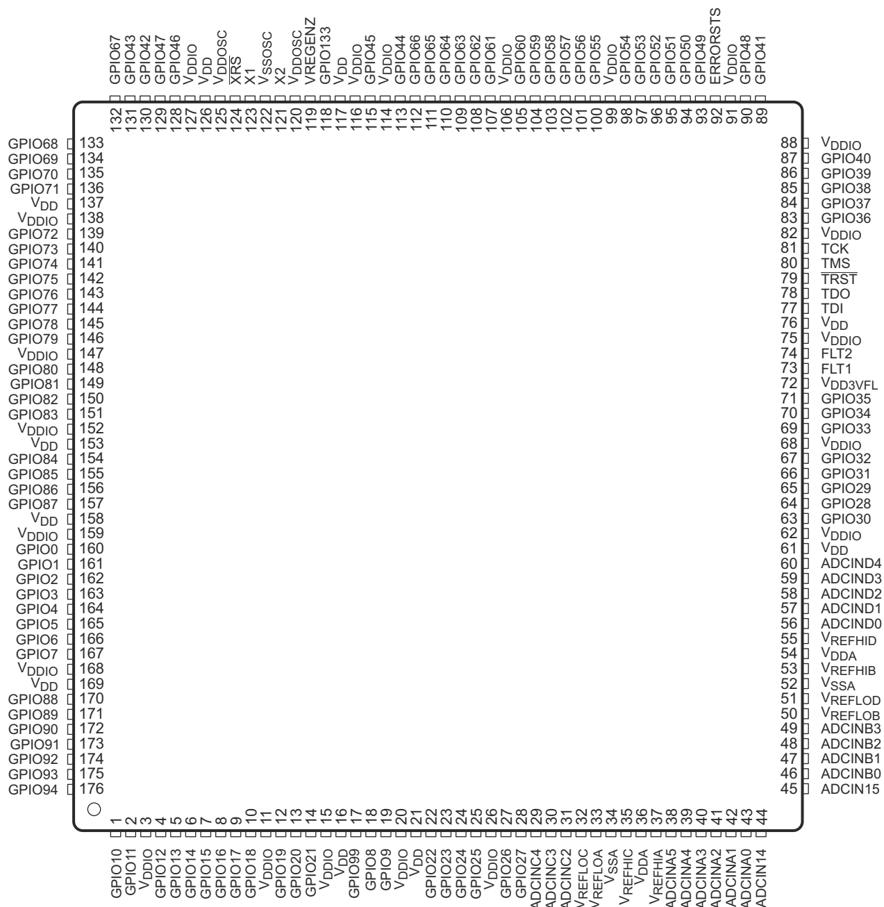
図 5-5. 176 ピン PTP PowerPAD 熱的に強化された薄型クワッドフラットパック (上面図)
