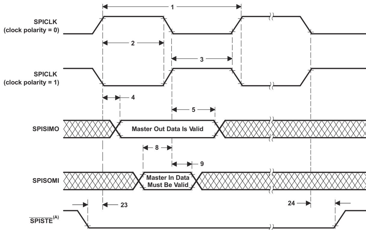
図 6-77. SPI マスタ モードの外部タイミング (クロック位相=0)
