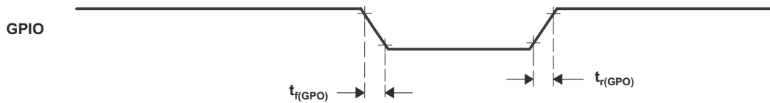
図 6-16. 汎用出力のタイミング
