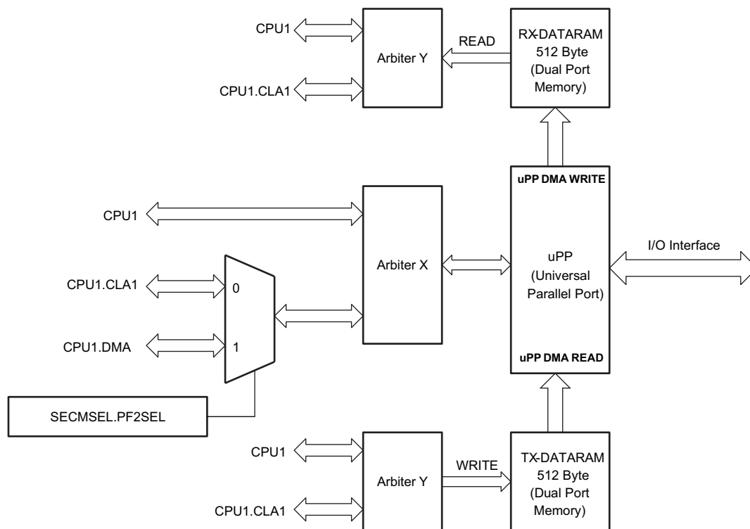
4-78. uPP Integration
