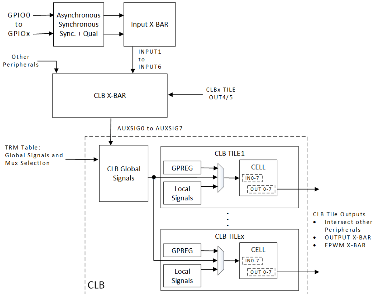
図 7-6. CLB の概要
