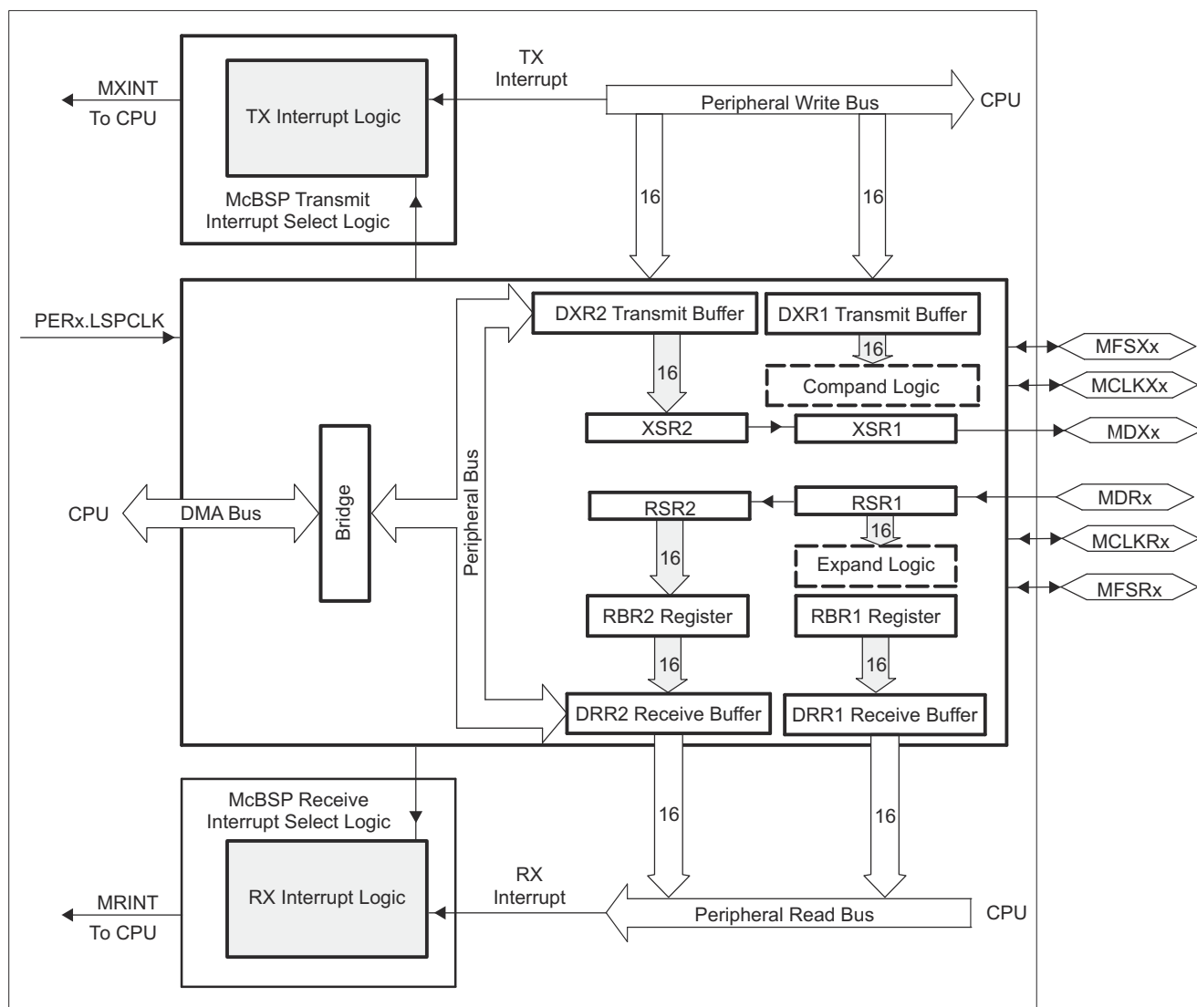
図 6-68. McBSP のブロック図
