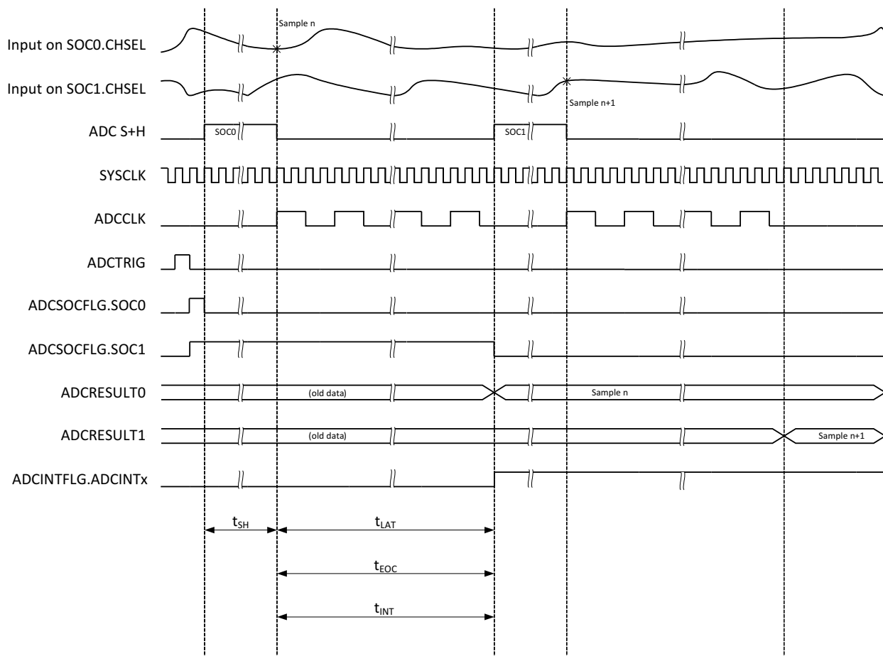
図 6-40. 16 ビット モードでの ADC タイミング
