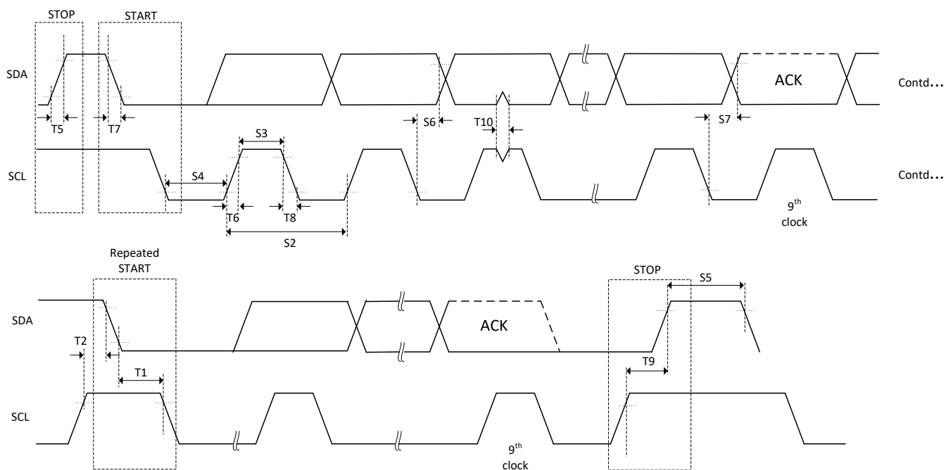
図 6-67. I2C タイミング図
