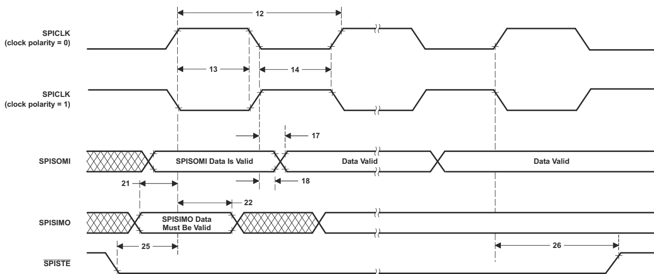
図 7-20. SPI スレーブ・モードの外部タイミング(クロック位相 = 1)
