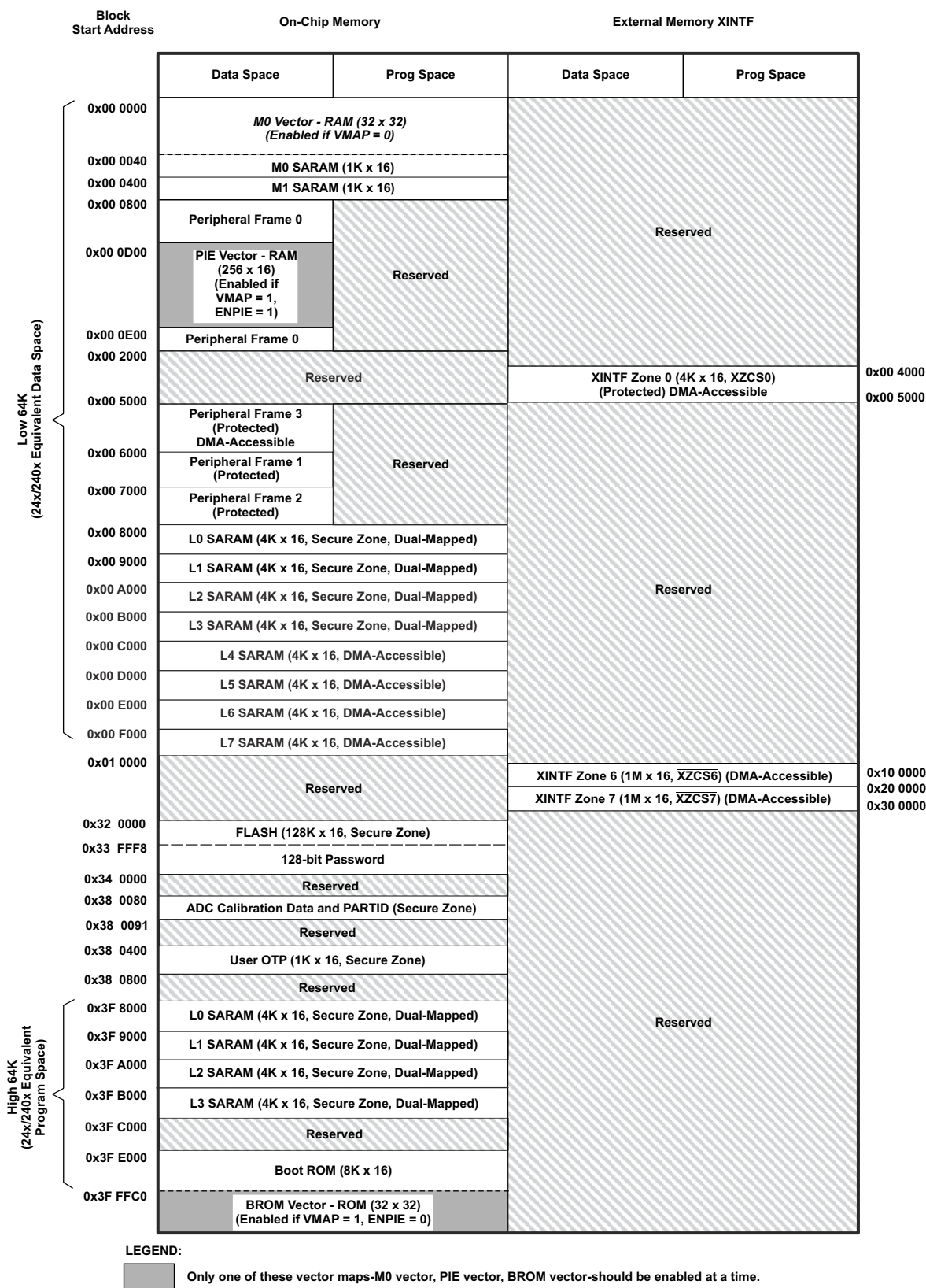
図 8-24. F28334、F28234 メモリ・マップ
