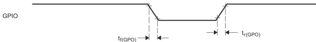
図 7-46. 汎用出力のタイミング
