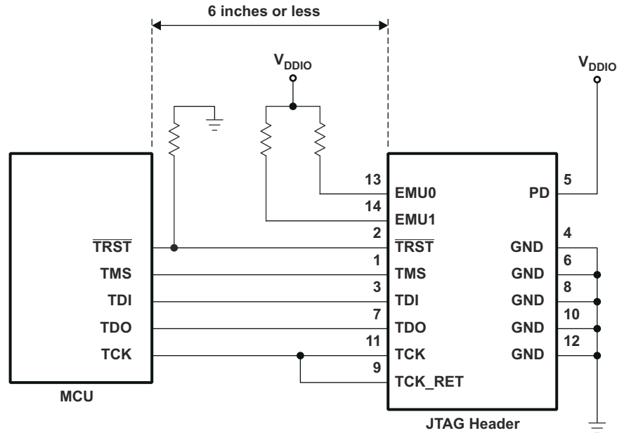
図 6-4. MCU との JTAG デバッグ プロローブ接続 (信号バッファリングなし)
