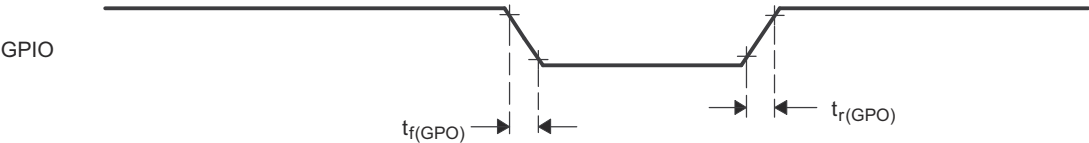
図 7-46. 汎用出力のタイミング
