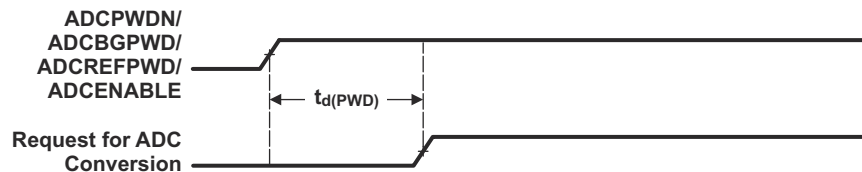
図 7-19. ADC 変換タイミング
