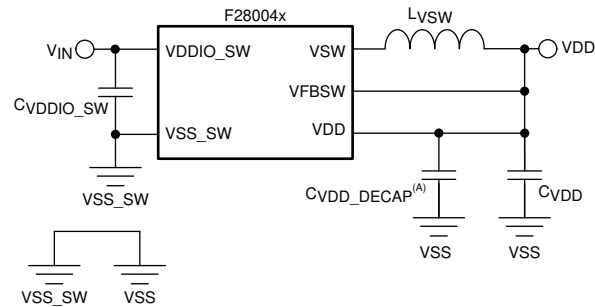
図 7-8. DC-DC 回路図
