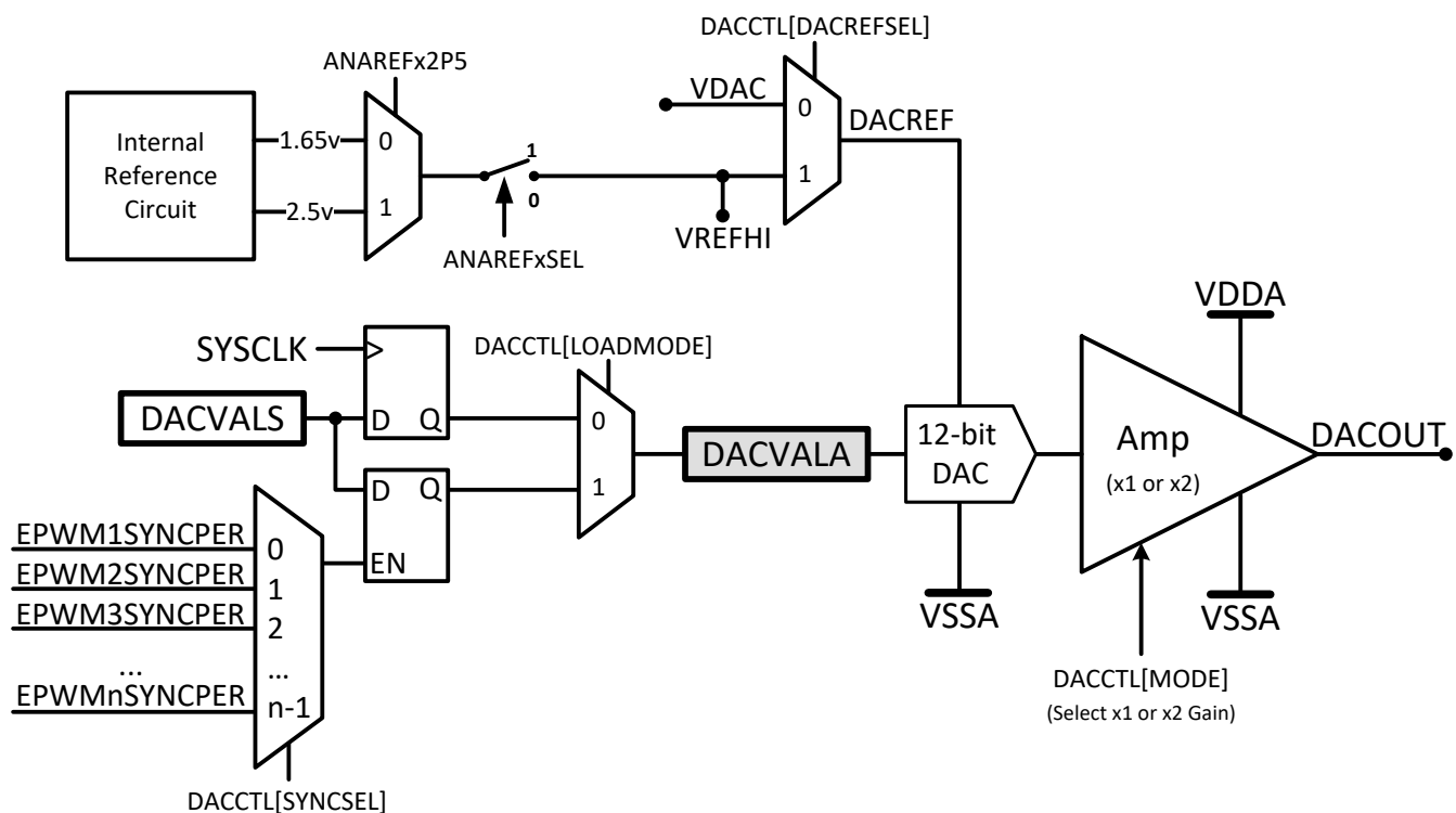
図 7-47. DAC モジュールのブロック図
