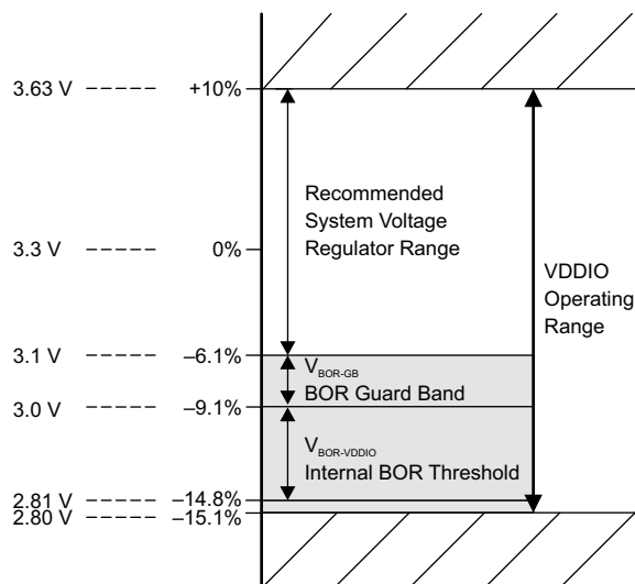
図 7-7. I/O BOR 動作領域
