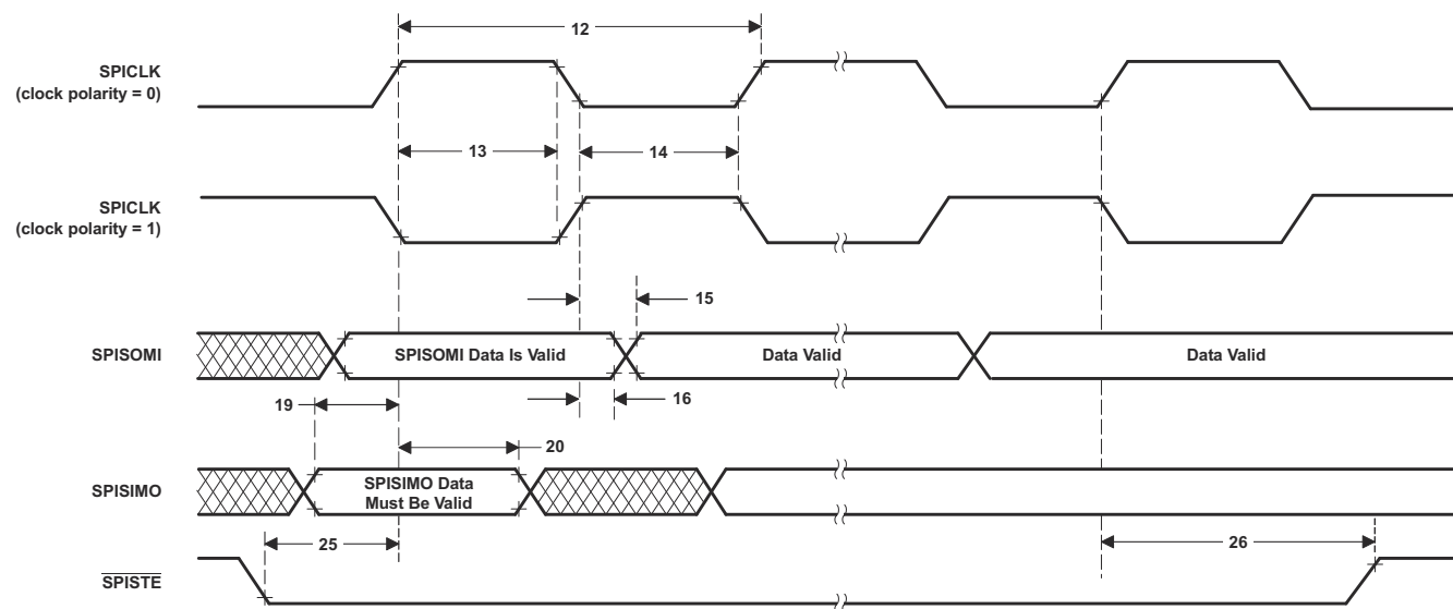
図 7-91. 高速 SPI スレーブ・モードの外部タイミング (クロック位相 = 1)
