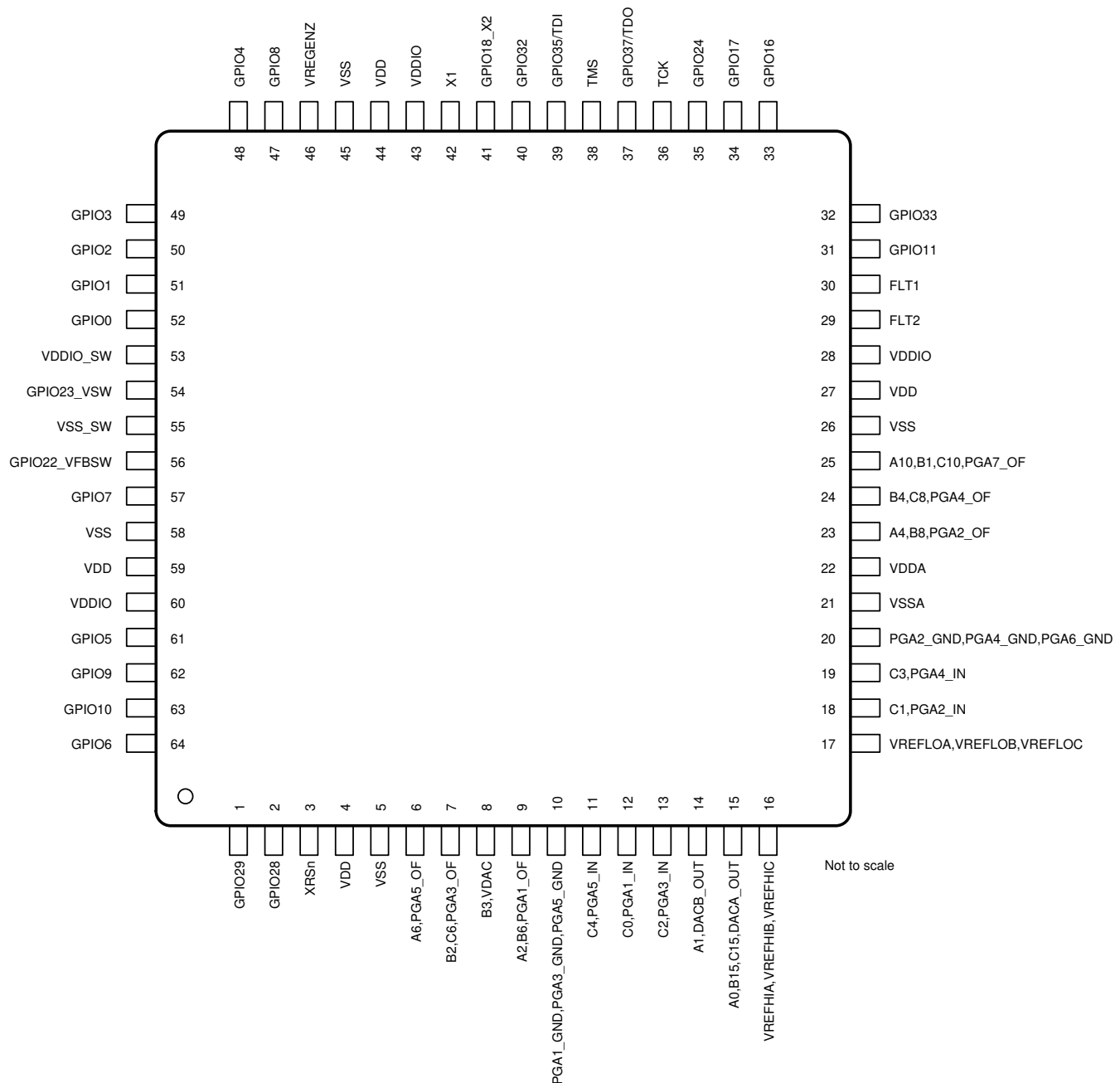
図 6-3. F280048/C、F280040/C 64 ピン PM 薄型クワッド・フラットバック - Q 温度 (上面図)
