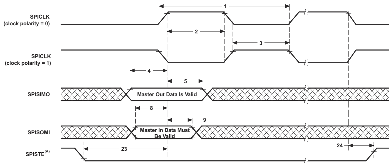
図 7-89. 高速 SPI マスタ・モードの外部タイミング (クロック位相 = 1)
