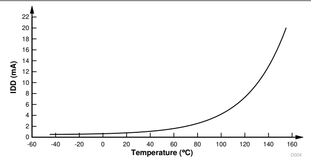
図 7-5. ホールド時の電流と温度 (°C) との関係
