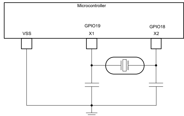
図 6-17. 外部水晶振動子
