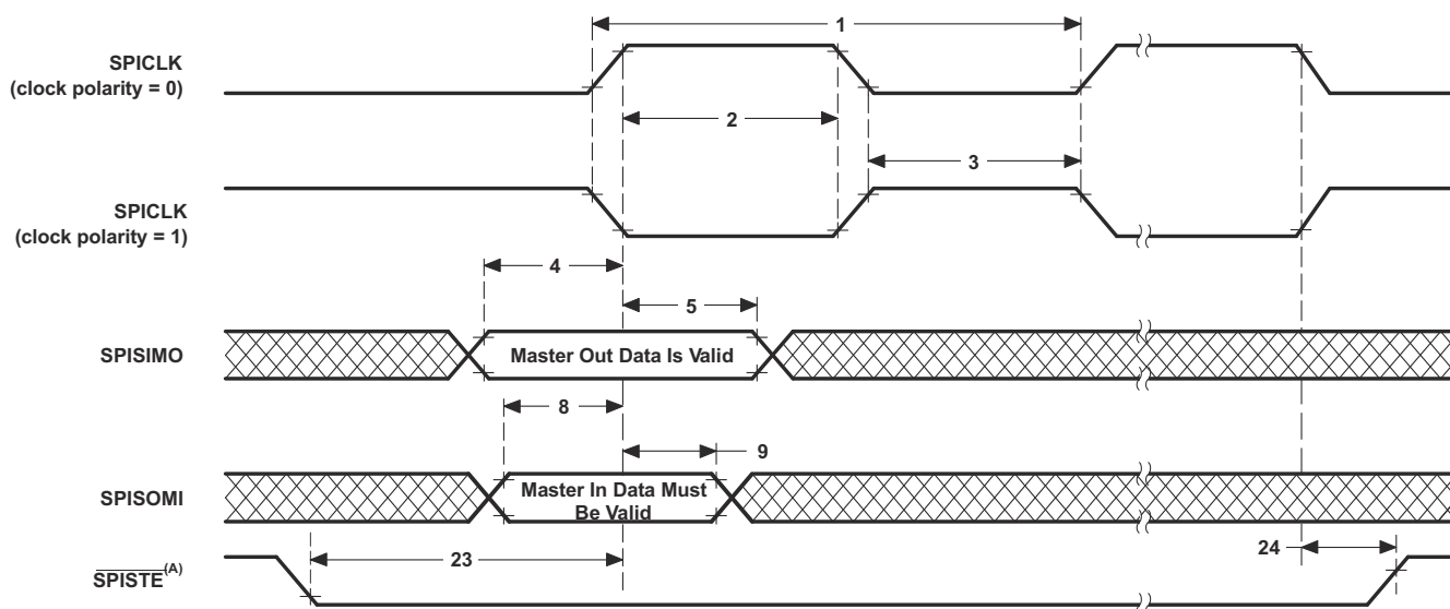
図 6-68. SPI マスタ・モードの外部タイミング (クロック位相 = 0)
