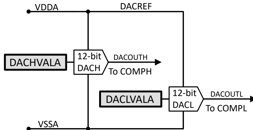
図 6-46. リファレンス DAC のブロック図
