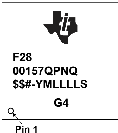
図 9-3. PN パッケージのパッケージ マーキング (AEC-Q100 グレード 1 認定)
