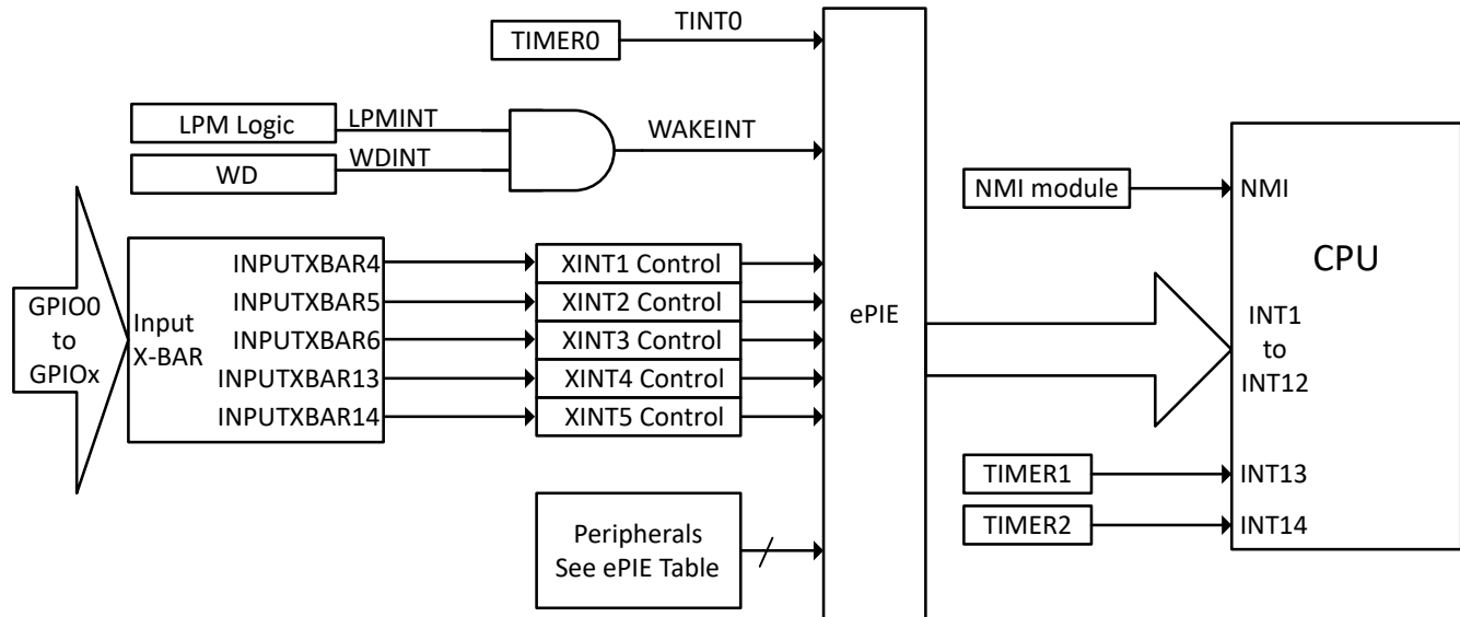
図 6-29. デバイス割り込みアーキテクチャ
