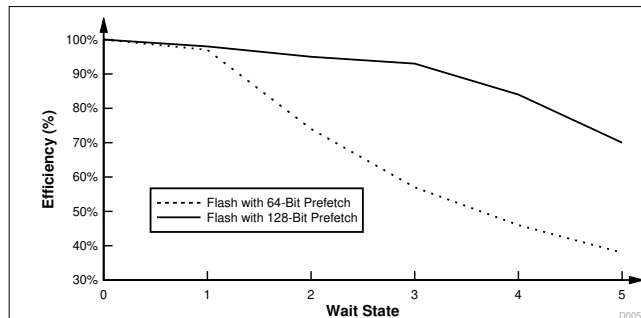
図 6-20. 多数の 32 ビット浮動小数点演算命令を含むアプリケーション・コード
