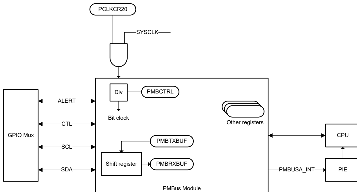
図 6-65. PMBus のブロック図
