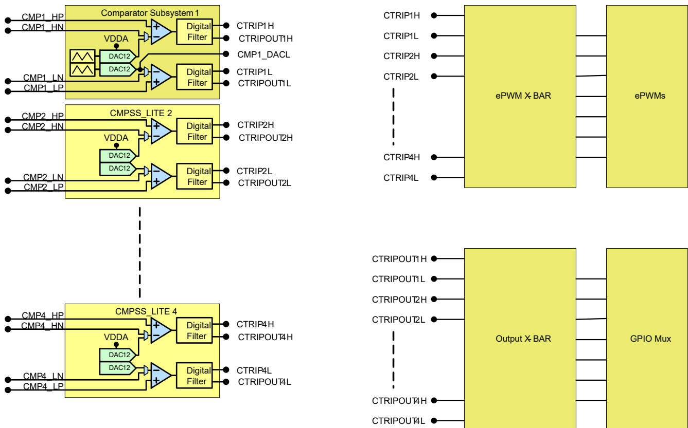
図 6-43. CMPSS の接続
