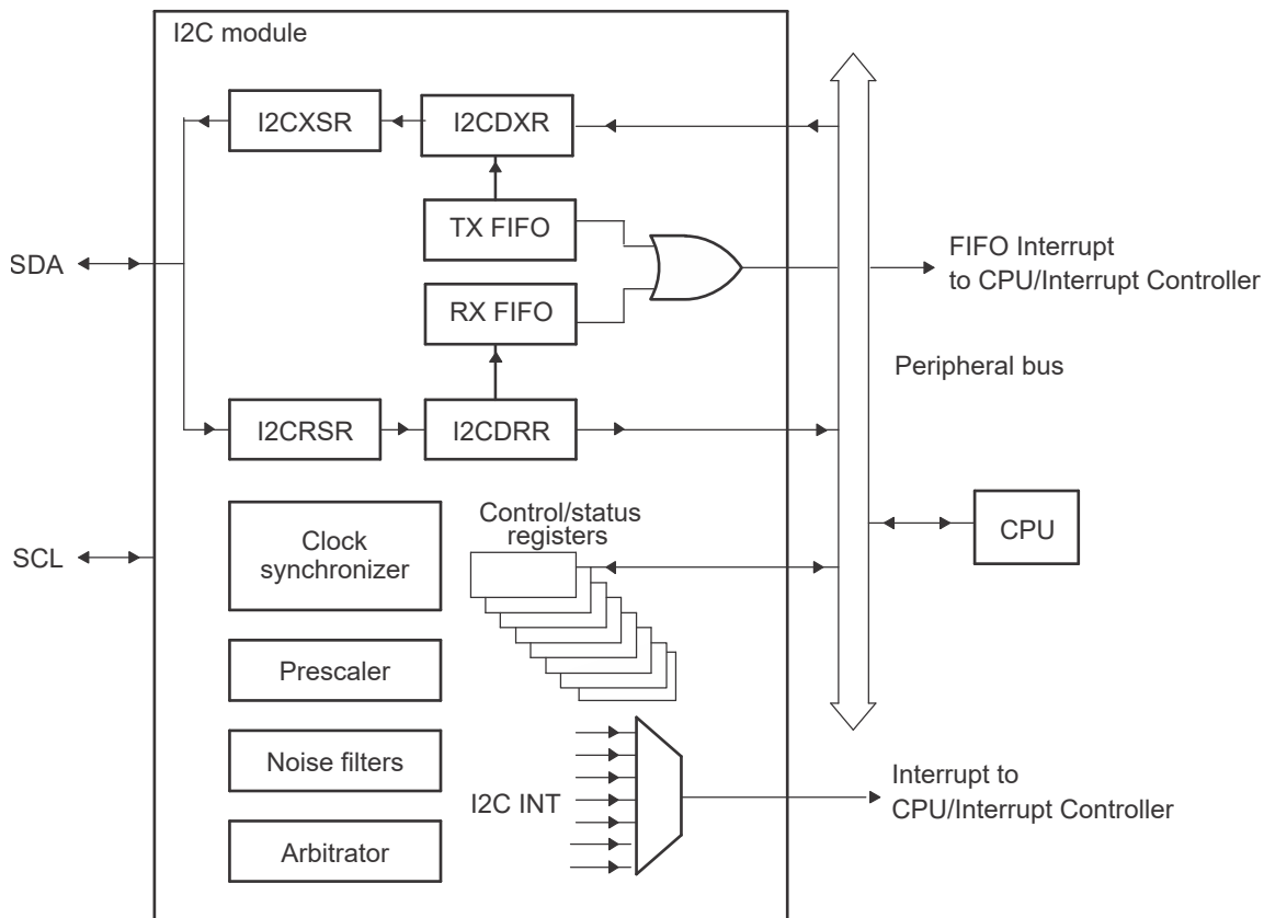
図 6-63. I2C ペリフェラル モジュール インターフェイス
