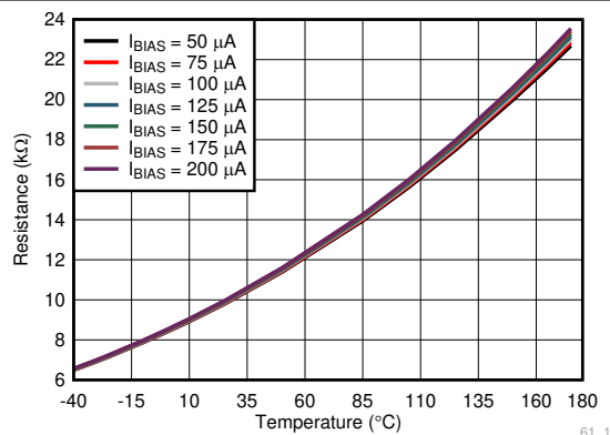
図 6-1. 車載グレード 0 の抵抗値と周囲温度との関係 (各種バイアス電流)
