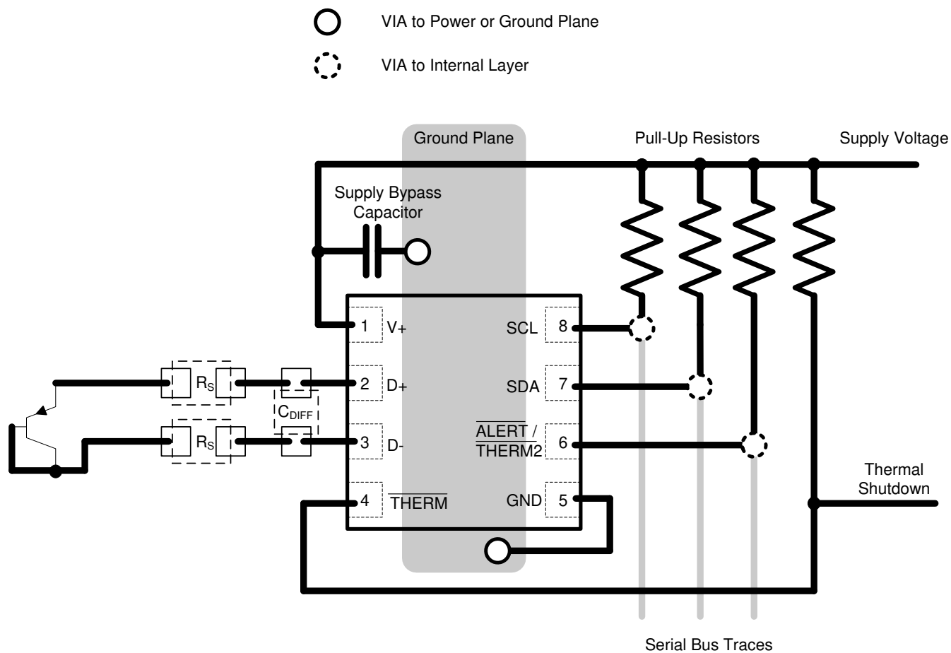
FIG 10-2. TMP451-Q1 Layout Example
