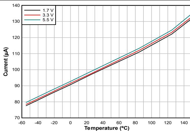
図 7-8. 温度変換電流と温度との関係
