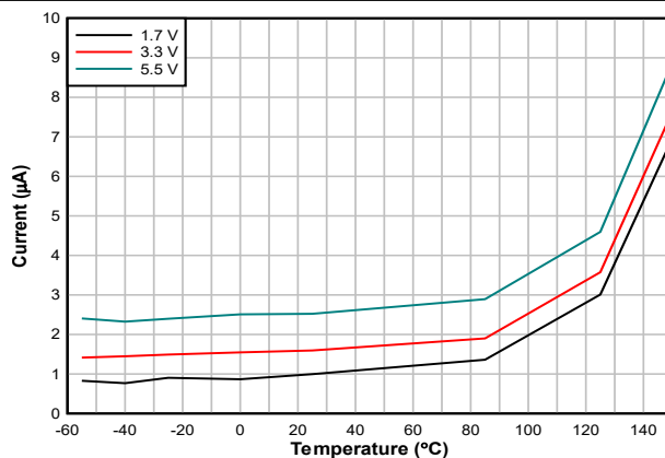
図 7-10. スタンバイ電流と温度との関係
