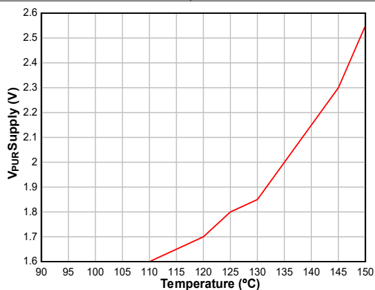
図 7-17. V_{PUR} 代表的な標準速度モード電源電圧と温度との関係
