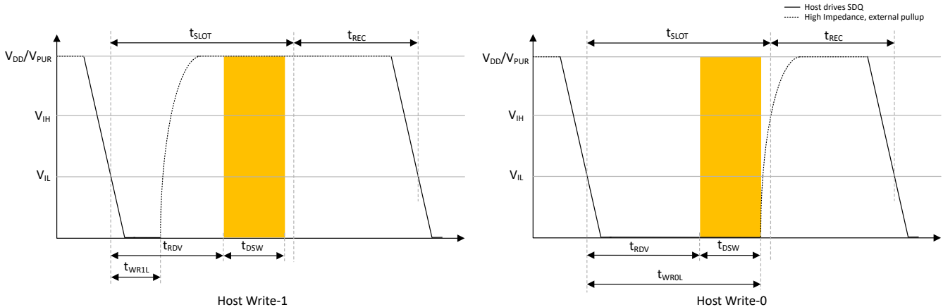
図 8-10. ホスト書き込み、デバイス読み取り
