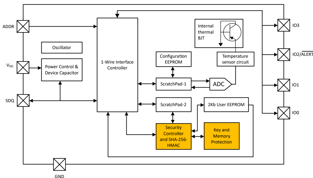
図 8-1. 機能ブロック図
