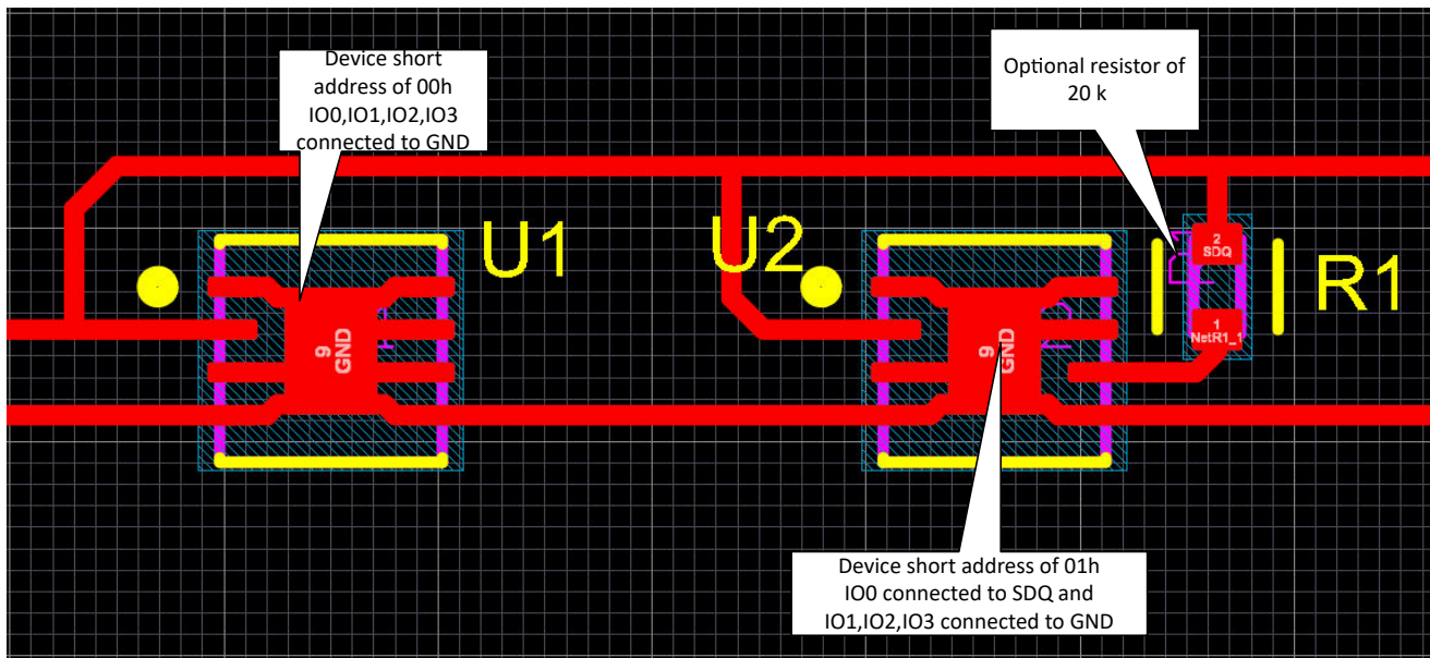
図 9-6. バス・パワー・モードでの IO ハードウェア・アドレス
