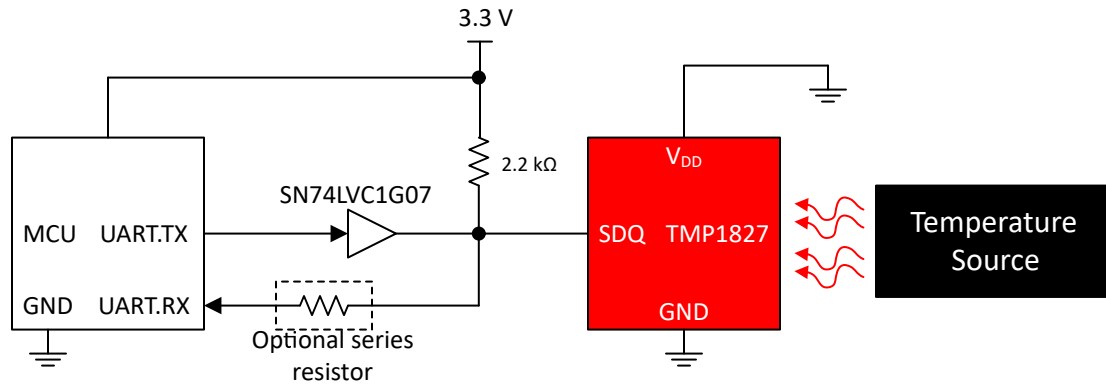
図 9-3. UART を使用したインターフェイス TMP1827
