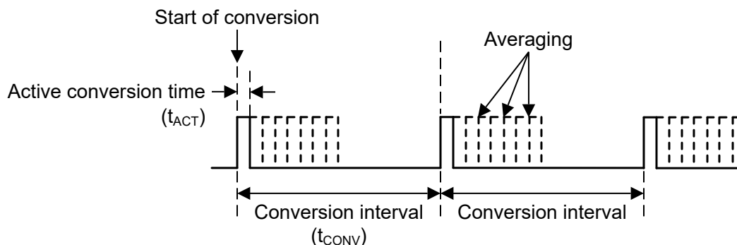
図 8-16. 連続変換モード
