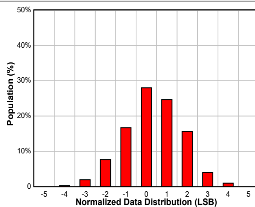
図 7-12. 変換時間 3ms、平均化オンでのデータの分散 (16 ビット・フォーマット)
