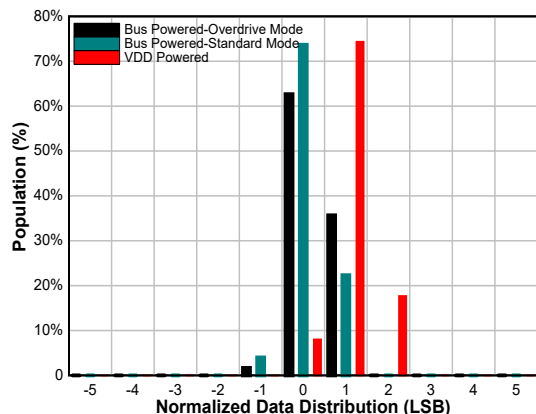
図 7-15. パワー・モードとバス速度のデータ分配
