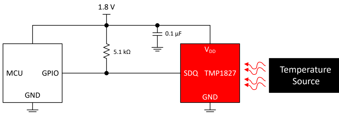
図 9-2. 電源モードのアプリケーション
