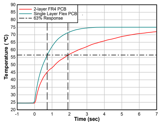
図 7-16. 熱応答時間 (NGR)
