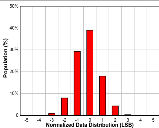
図 7-11. 変換時間 5.5ms、平均化オンでのデータの分散 (16 ビット・フォーマット)
