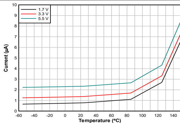
図 7-9. シャットダウン電流と温度との関係
