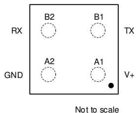
図 5-1. YFF および YBK パッケージ 4 ピン DSBGA (上面図)
