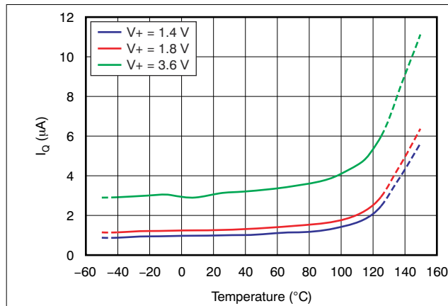
図 8-2. 代表的な静止電流と温度との関係
