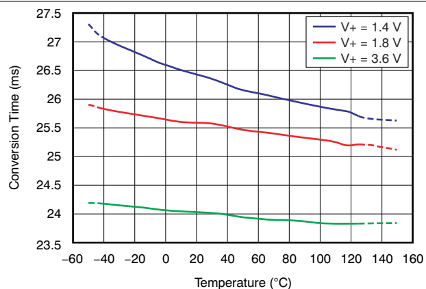
図 6-4. 変換時間と温度との関係
