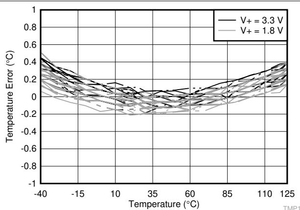
図 6-5. 温度誤差と温度との関係 (YFF パッケージ)
