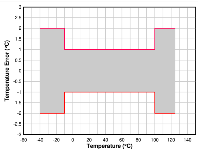
図 8-3. 温度誤差と温度との関係
