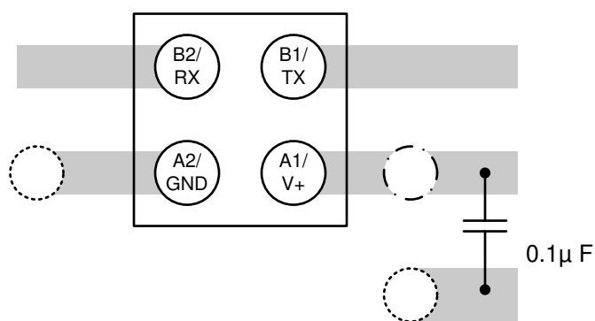
図 8-5. レイアウト例
