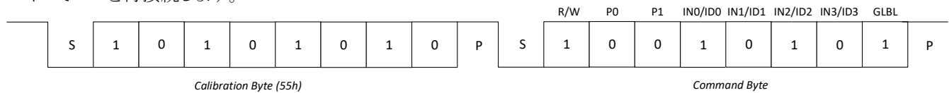
図 7-11. グローバル・クリア割り込みコマンドのフロー
