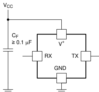
図 8-4. バイパス・コンデンサによる電源ノイズの低減
