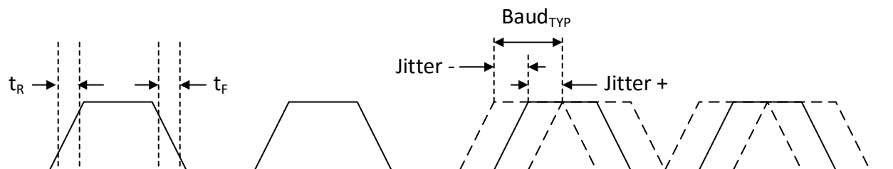
図 6-1. SMAART Wire™/UART インターフェイスのタイミング図
