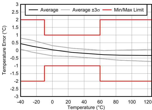
図 6-4. TMP1075NDRL の温度誤差と温度との関係
