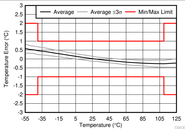
図 6-2. DGK and D の温度誤差と温度との関係
