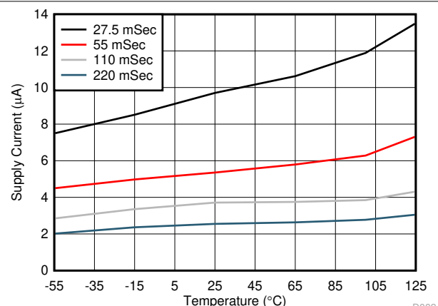
図 6-6. 平均電流と変換レートおよび温度との関係
