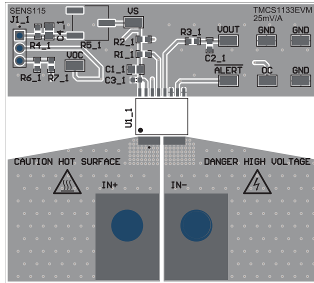
図 9-5. 推奨されるボードレイアウト
