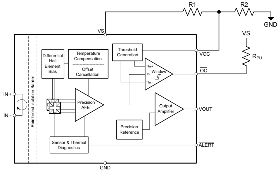
図 8-6. 電源電圧を使用して、過電流スレッシュホールドをユーザーが設定可能
