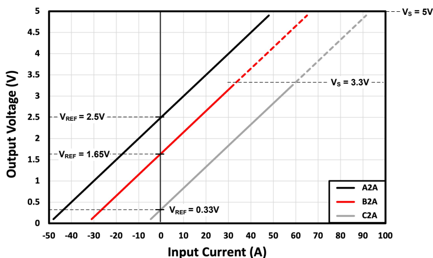
図 8-5. TMCS11xxx2A の出力電圧と入力電流との関係
