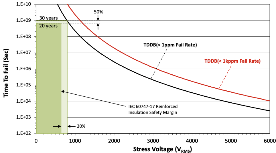
図 8-2. 絶縁寿命
