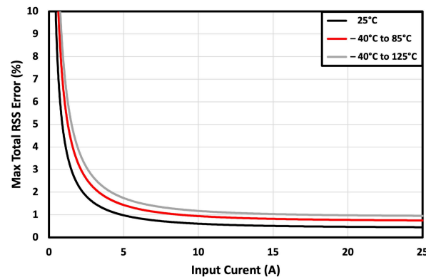
図 9-1. RSS Error vs Input Current
