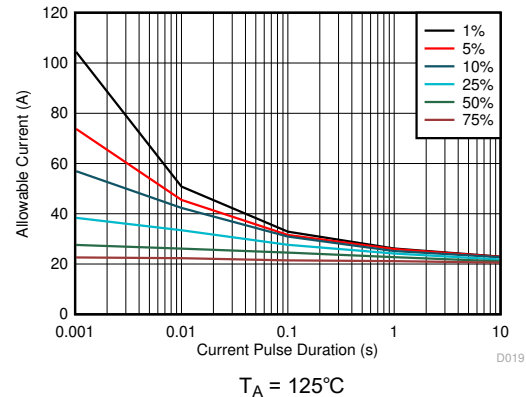
図 7-9. 最大反復パルス電流とパルス期間との関係
