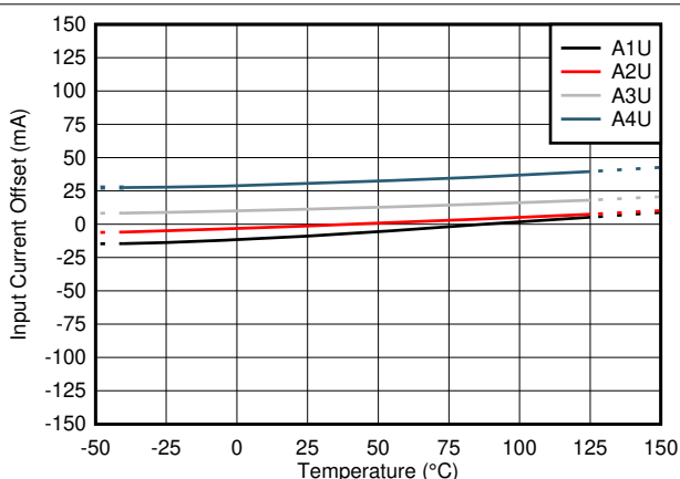
図 6-4. TMCS1101AxU-Q1 の入力オフセット電流と温度との関係
