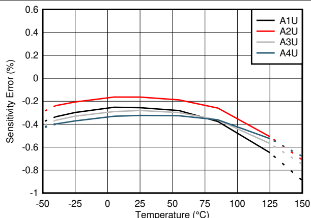
図 6-2. TMCS1101AxU-Q1 の感度誤差と温度との関係
