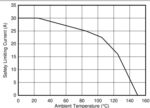
図 6-28. 安全性制限電流による熱特性低下曲線、サイド 1
