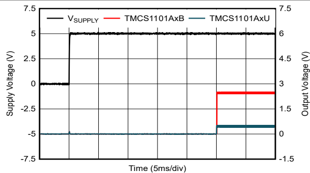
図 6-26. スタートアップ過渡応答
