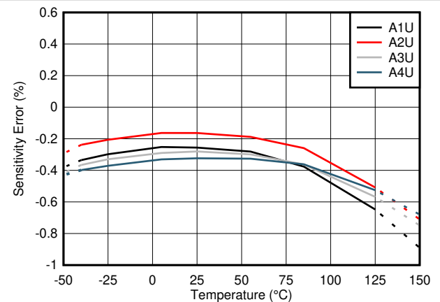
図 8-5. 温度範囲全体での感度ドリフト (U バリエーション)
