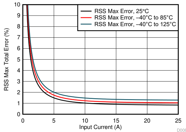
図 9-1. RSS 誤差と入力電流との関係
