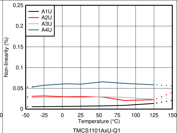
図 6-6. 非線形性線性と温度との関係
