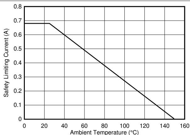
図 6-29. 安全性制限電流による熱特性低下曲線、サイド 2
