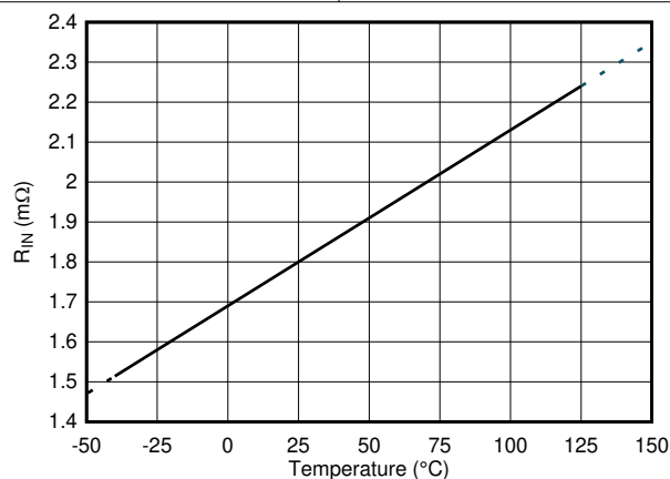
図 6-27. 入力導体の抵抗と温度との関係
