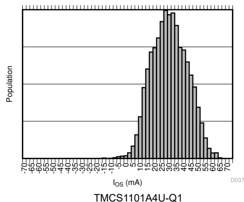
図 6-16. 入力オフセット電流の製品分布
