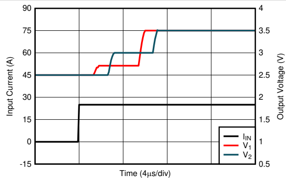
図 6-23. 電圧出カステップ、立ち上がり
