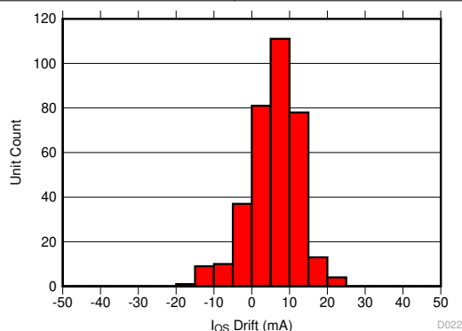
図 8-8. AEC-Q100 高温動作寿命ストレス テスト後の入力換算オフセット ドリフト
