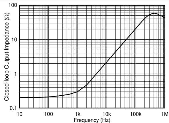
図 6-20. 出力インピーダンス 対 周波数
