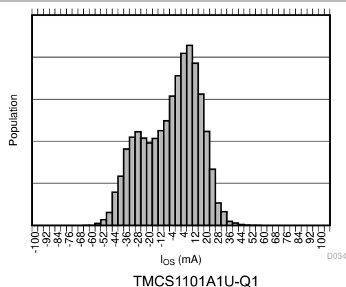
図 6-10. 入力オフセット電流の製品分布
