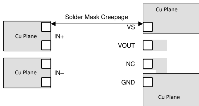
図 9-5. システムの沿面距離要件を満たすレイアウト
