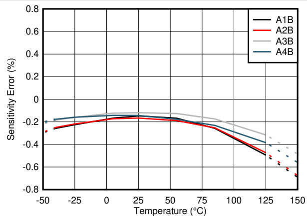
図 8-4. 温度範囲全体での感度ドリフト (B バリエーション)
