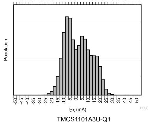
図 6-14. 入力オフセット電流の製品分布
