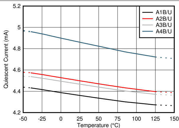
図 6-21. 静止電流と温度との関係
