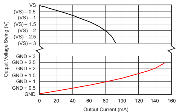
図 6-19. 出力スイングと出力電流との関係
