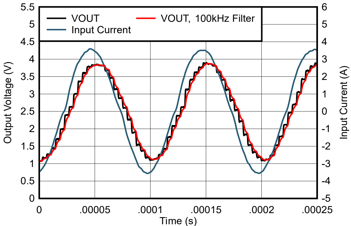
図 8-11. 10kHz の正弦波入力電流に対する応答動作
