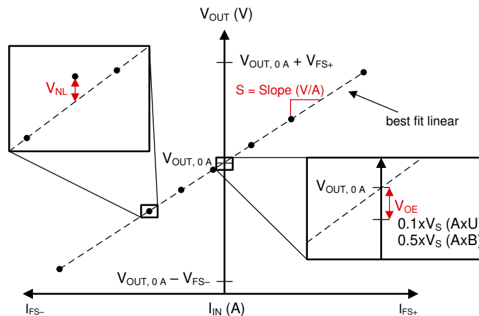
図 7-1. 感度、オフセット、非直線性誤差
