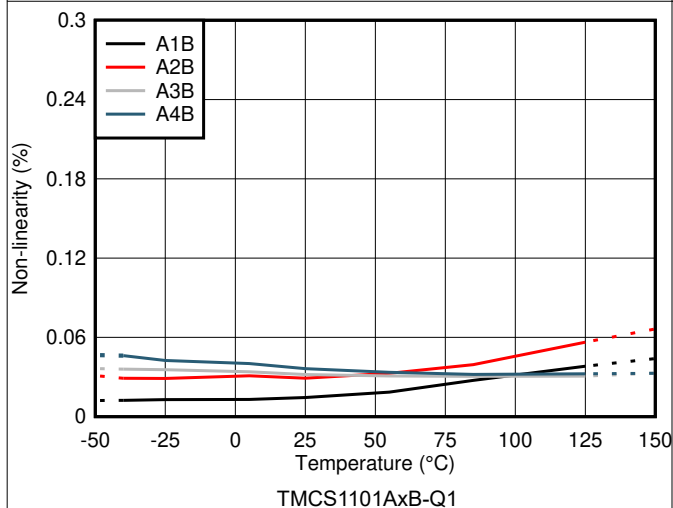
図 6-5. 非線形性線性と温度との関係
