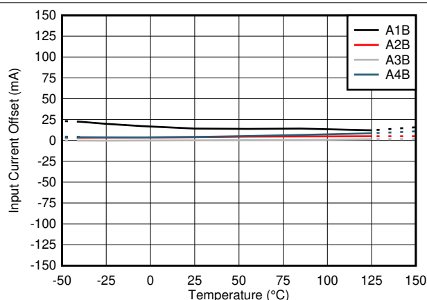
図 6-3. TMCS1101AxB-Q1 の入力オフセット電流と温度との関係
