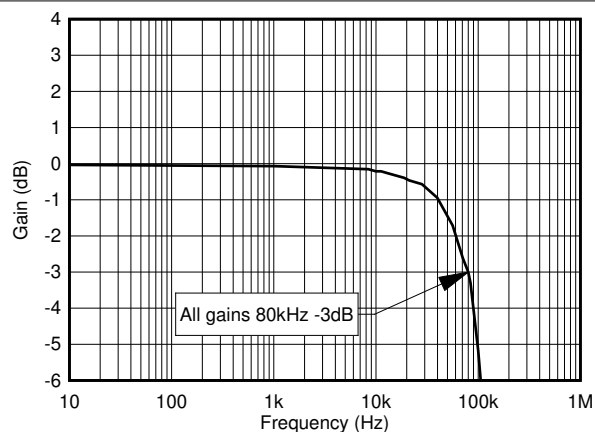
図 6-17. 感度と周波数との関係、すべてのゲインは 1Hz に正規化
