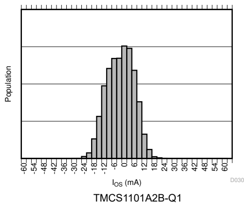
図 6-11. 入力オフセット電流の製品分布
