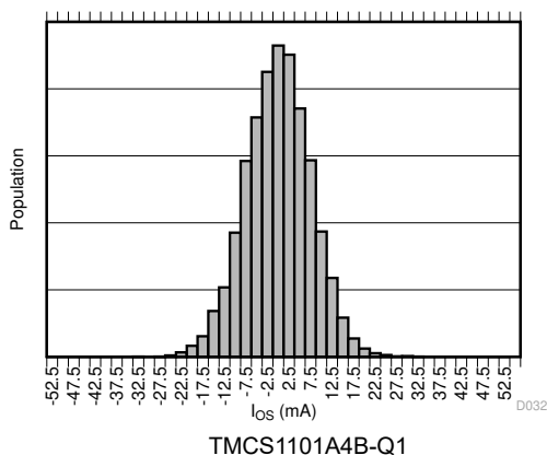
図 6-15. 入力オフセット電流の製品分布
