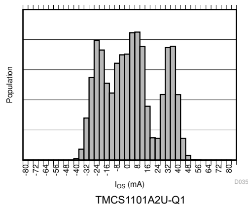
図 6-12. 入力オフセット電流の製品分布
