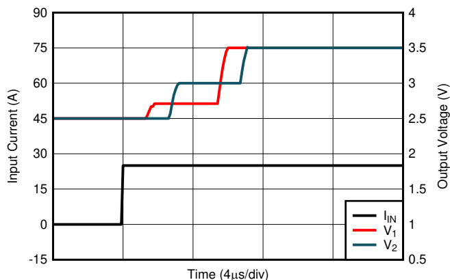
図 8-12. 1V の出力スイングに十分な入力電流ステップに対しての過渡応答
