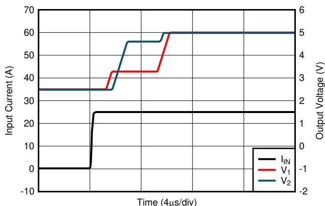
図 8-13. 大きな入力電流ステップに対する過渡応答
