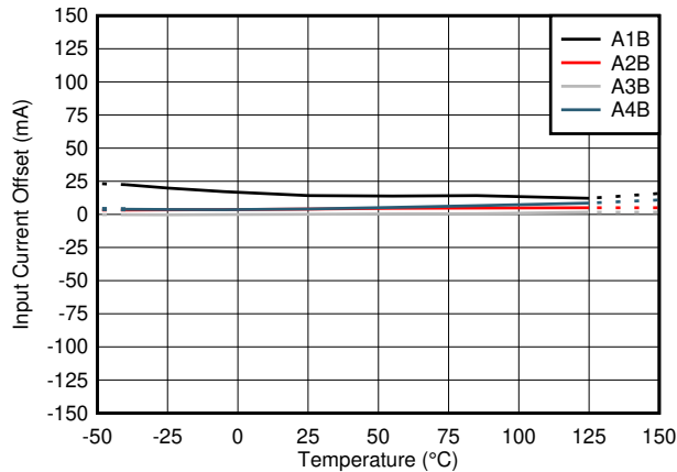
図 8-2. 温度範囲全体にわたるオフセット誤差ドリフト (B バリエーション)
