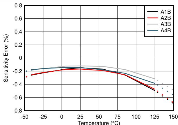
図 6-1. TMCS1101AxB-Q1 の感度誤差と温度との関係
