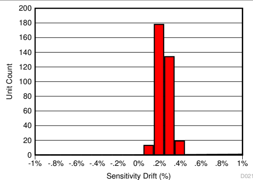
図 8-7. AEC-Q100 高温動作寿命ストレス テスト後の感度誤差ドリフト
