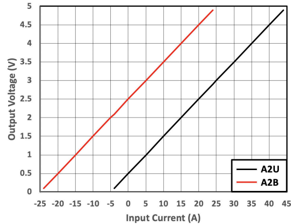
図 8-14. TMCS1101A2B-Q1 および TMCS1101A2U-Q1 の出力電圧と入力電流の関係
