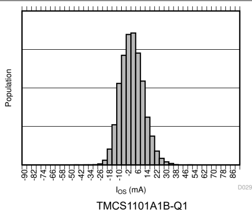
図 6-9. 入力オフセット電流の製品分布
