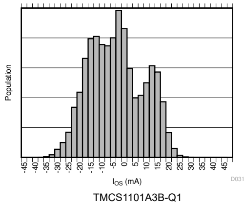
図 6-13. 入力オフセット電流の製品分布
