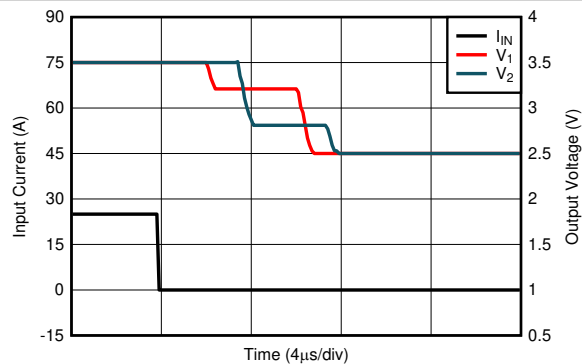
図 6-24. 電圧出カステップ、立ち下がり
