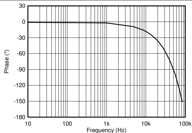
図 6-18. 位相と周波数との関係、すべてのゲイン
