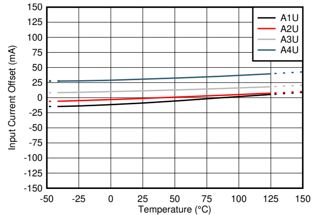
図 8-3. 温度範囲全体にわたるオフセット誤差ドリフト (U バリエーション)
