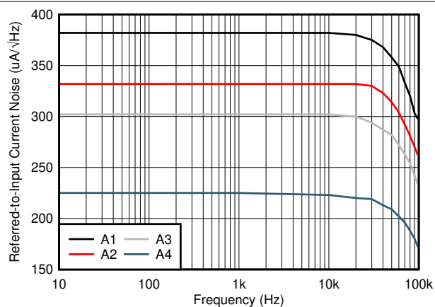
図 6-22. 入力換算ノイズと周波数との関係
