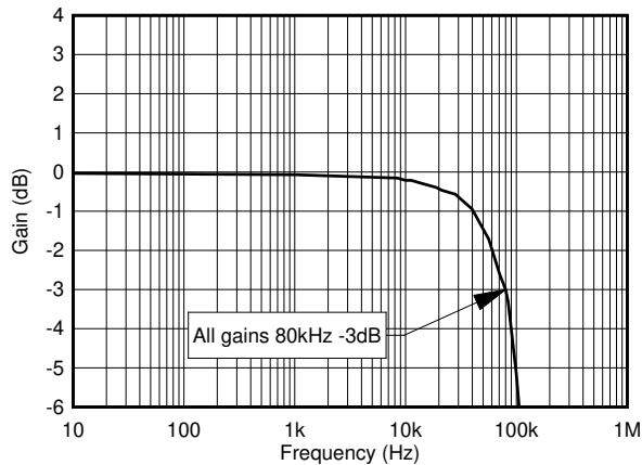
図 8-9. 正規化されたゲイン、すべてのバリエーション
