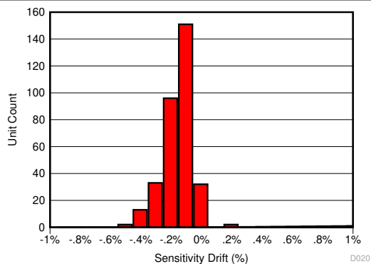
図 8-6. 130°C、85% RH HAST 後の感度誤差
