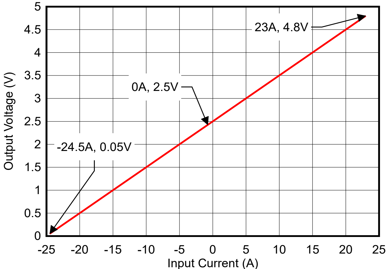
図 9-3. アプリケーションの設計伝達曲線の例
