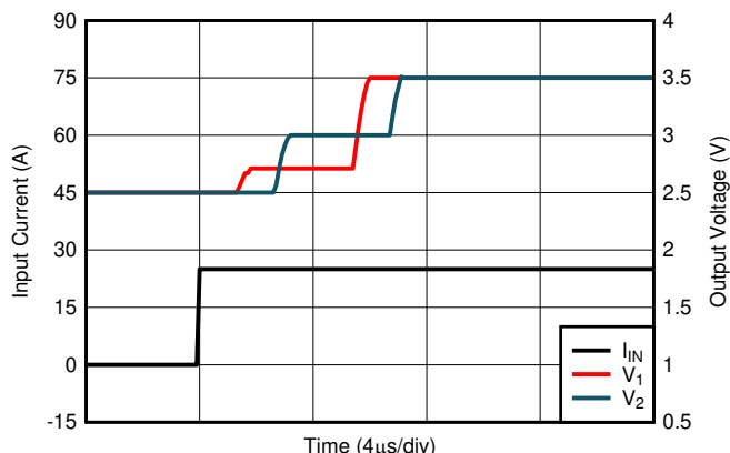
図 8-12. 1V の出力スイングに十分な入力電流ステップに対しての過渡応答
