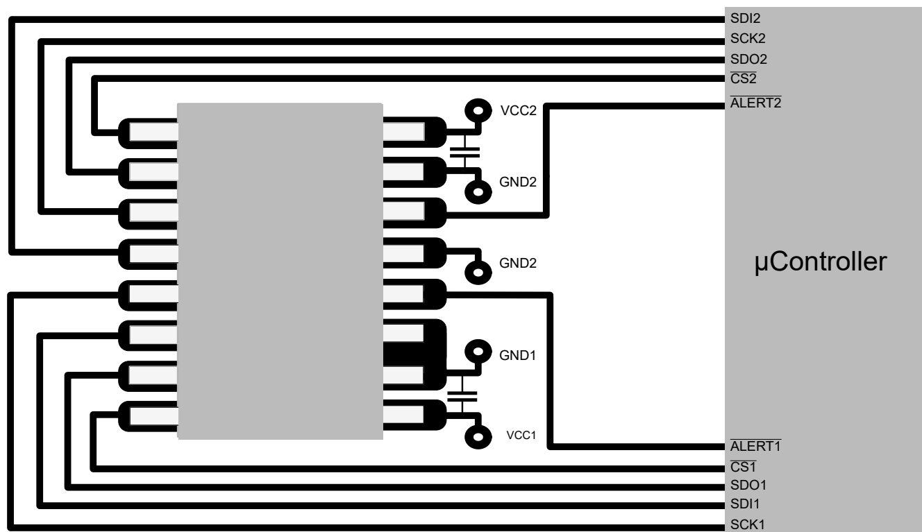
7-9. Layout Example With TMAG5170D-Q1
