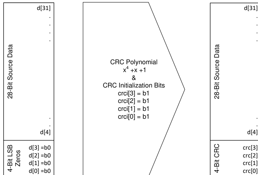
図 6-9. 4-Bit CRC Calculation
