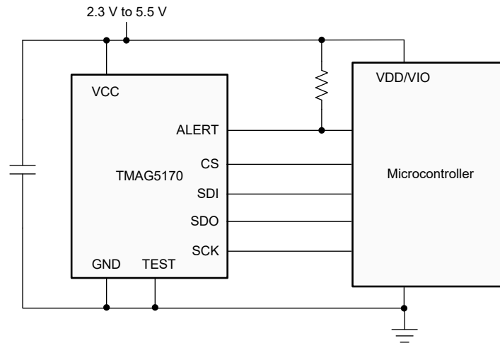
図 7-4. TMAG5170D-Q1 Application Diagram
