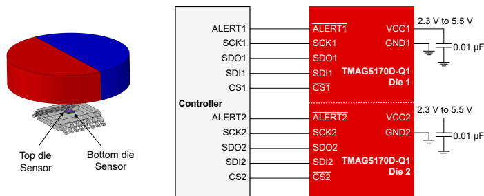
アプリケーションのブロック図
